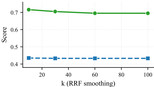
RRF: Effect of k Parameter
