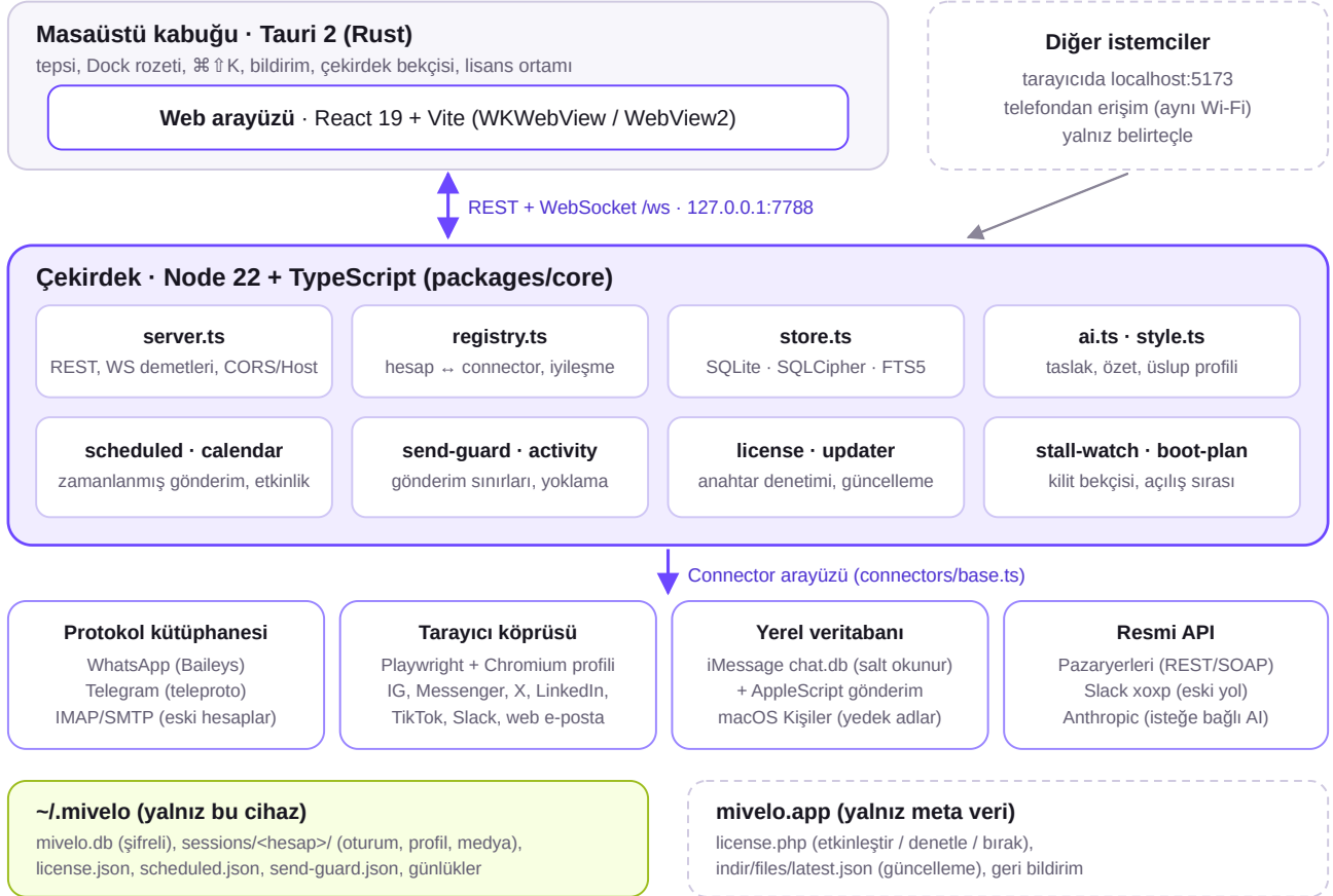
Şekil 1. Katmanlar ve veri akışı. Mesaj içeriği yalnız cihazda kalır; mivelo.app'e yalnız lisans, güncelleme denetimi ve kullanıcının gönderdiği geri bildirim gider.
