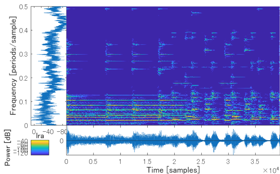
Fig. 2 残響時間 2.6 秒の観測音のスペクトログラム (SDR=-0.70 dB)
