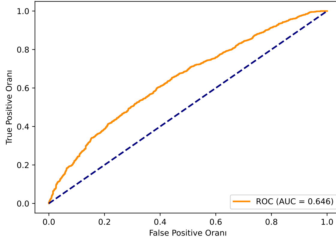
ROC Eğrisi
