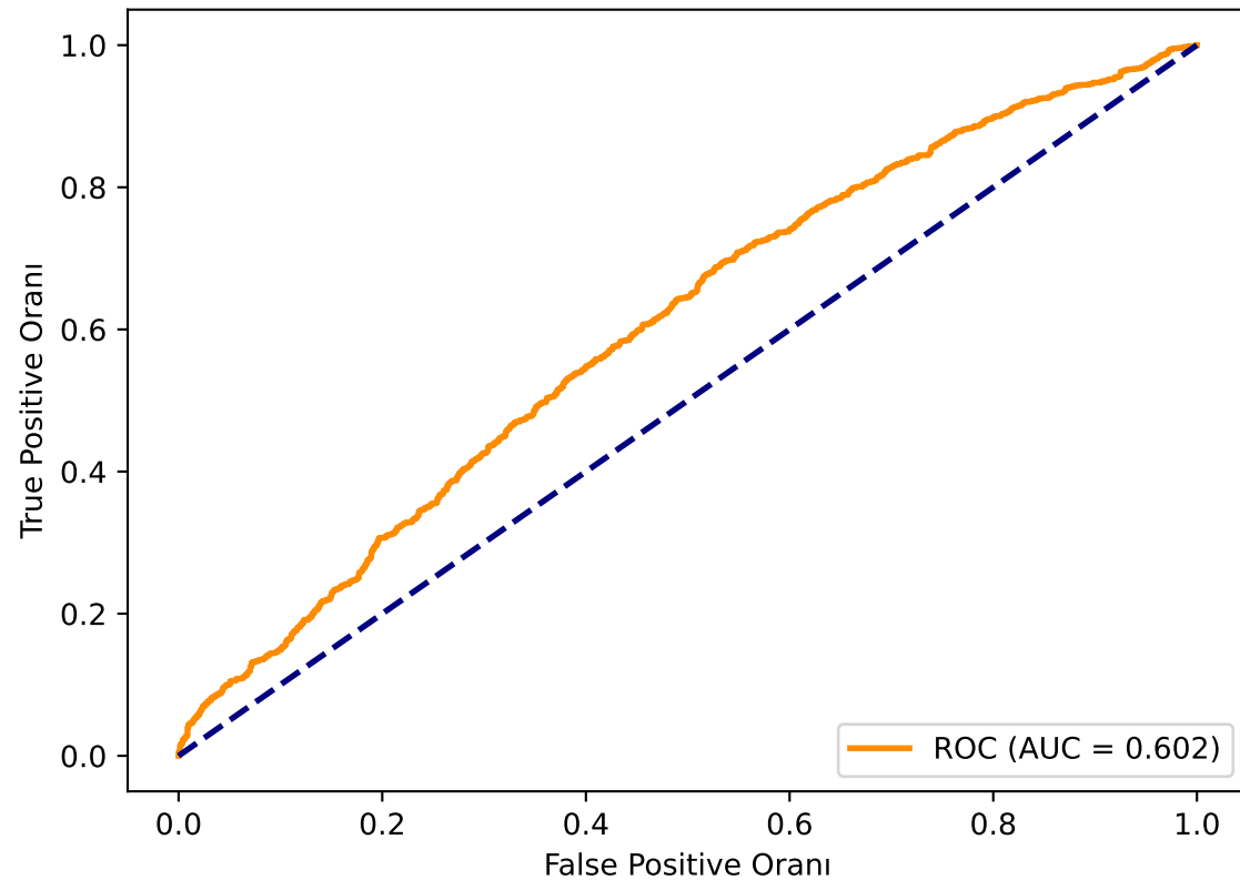
ROC Eğrisi
