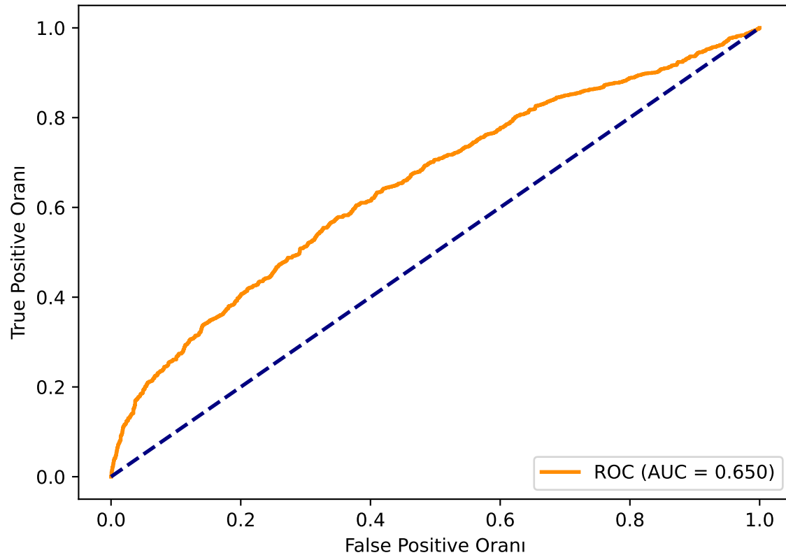
ROC Eğrisi
