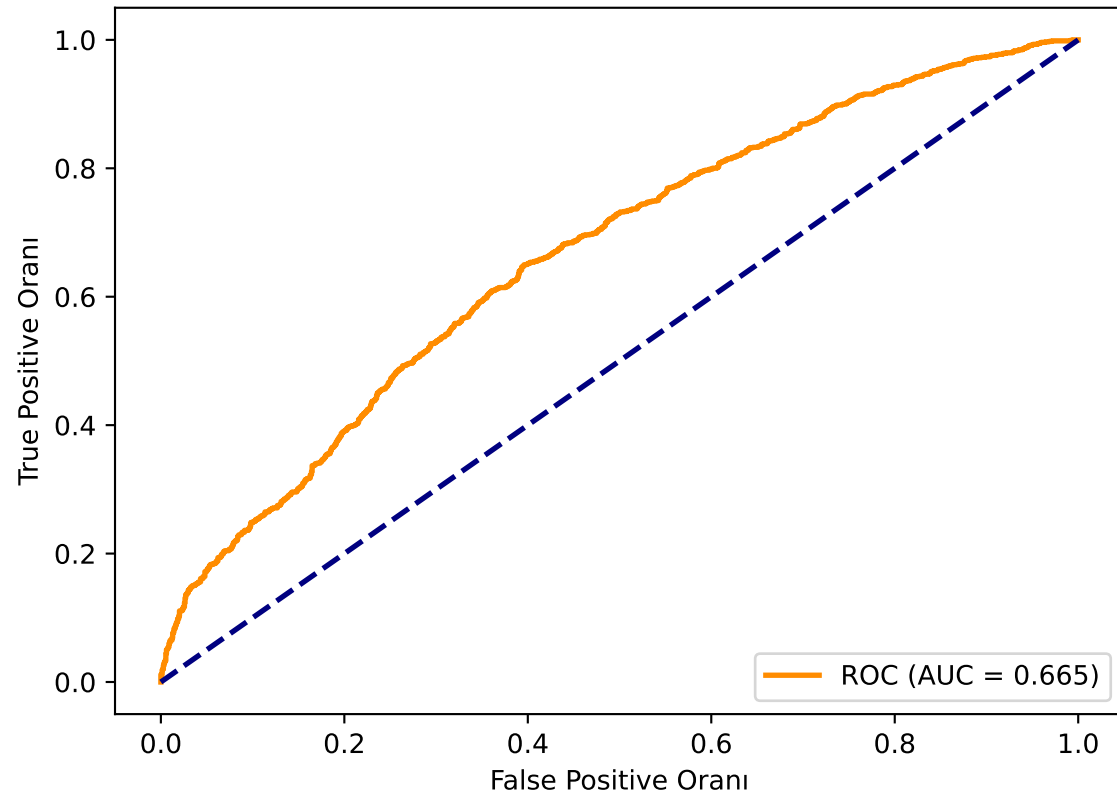
ROC Eğrisi
