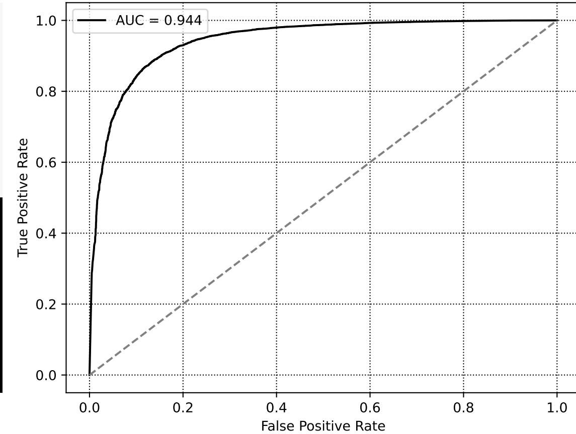
EXP004: ROC Eğrisi
