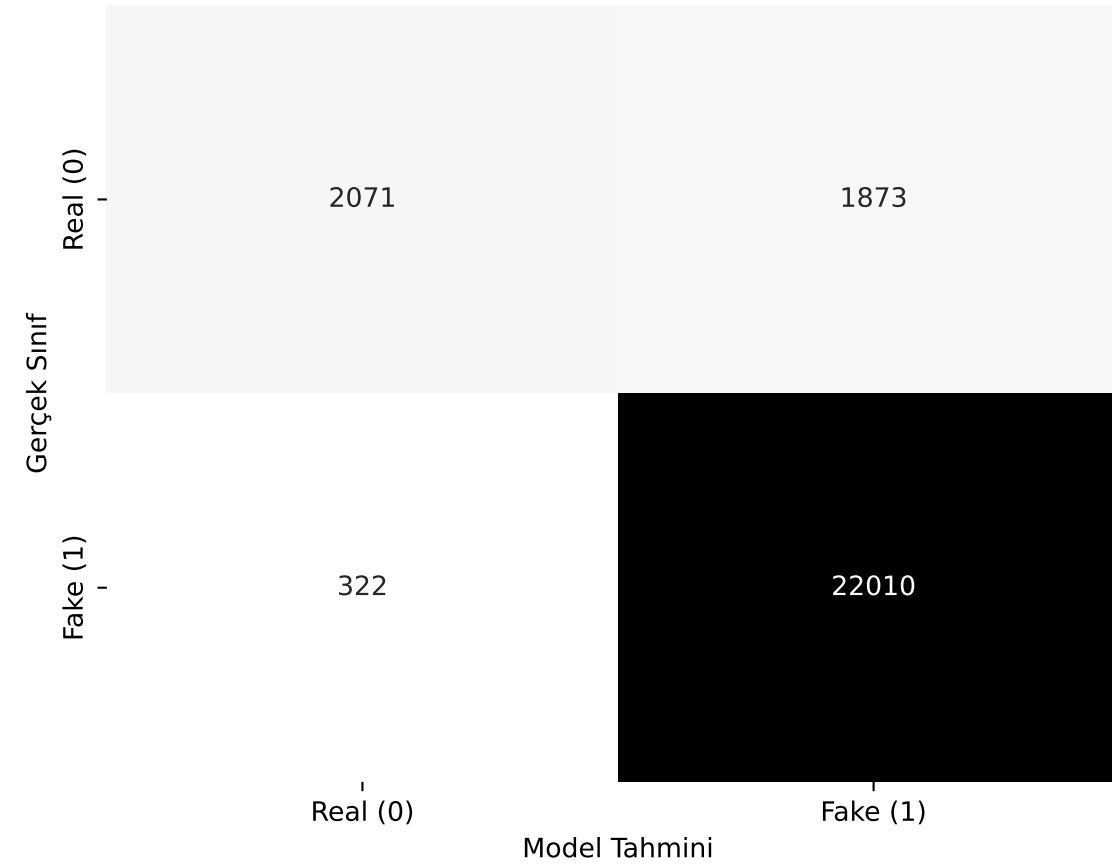
EXP004: Karmaşıklık Matrisi
