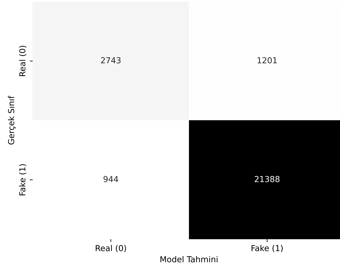
EXP001: Karmaşıklık Matrisi
