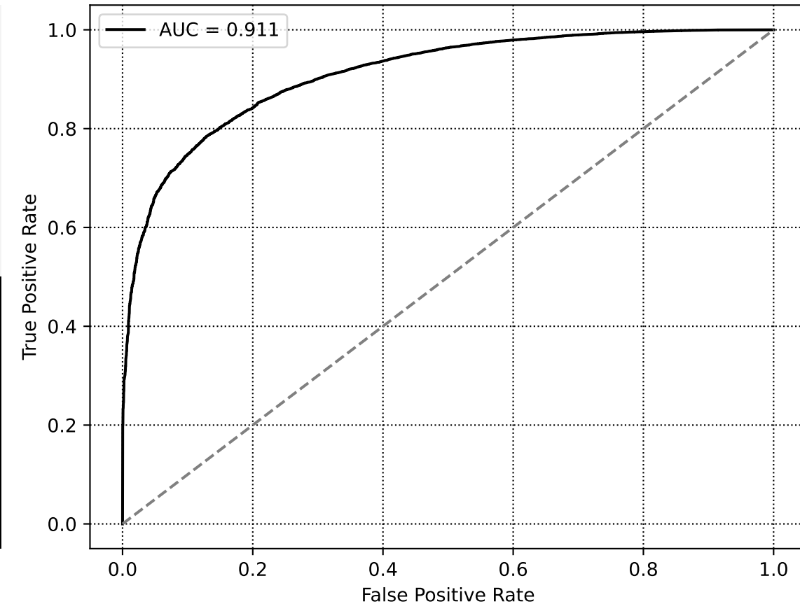
EXP002: ROC Eğrisi
