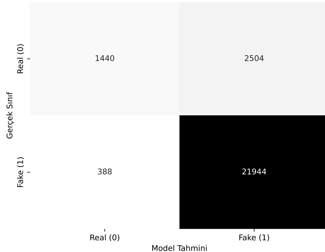
EXP002: Karmaşıklık Matrisi
