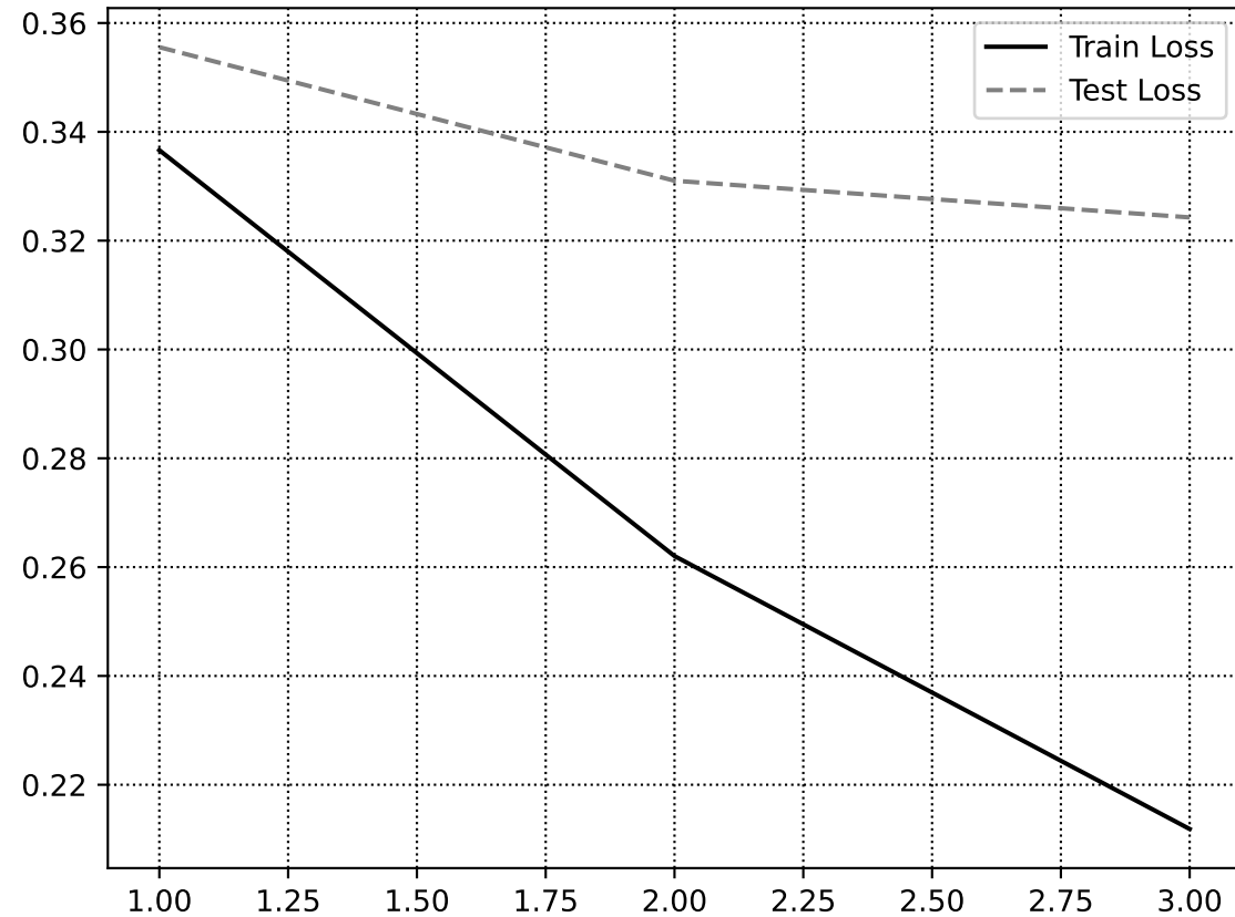
EXP002: Eğitim/Test Kayıp Eğrisi
