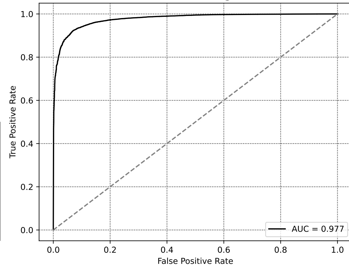
EXP005: ROC Eğrisi
