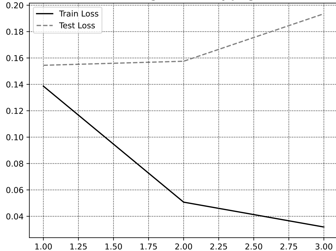
EXP005: Eğitim/Test Kayıp Eğrisi
