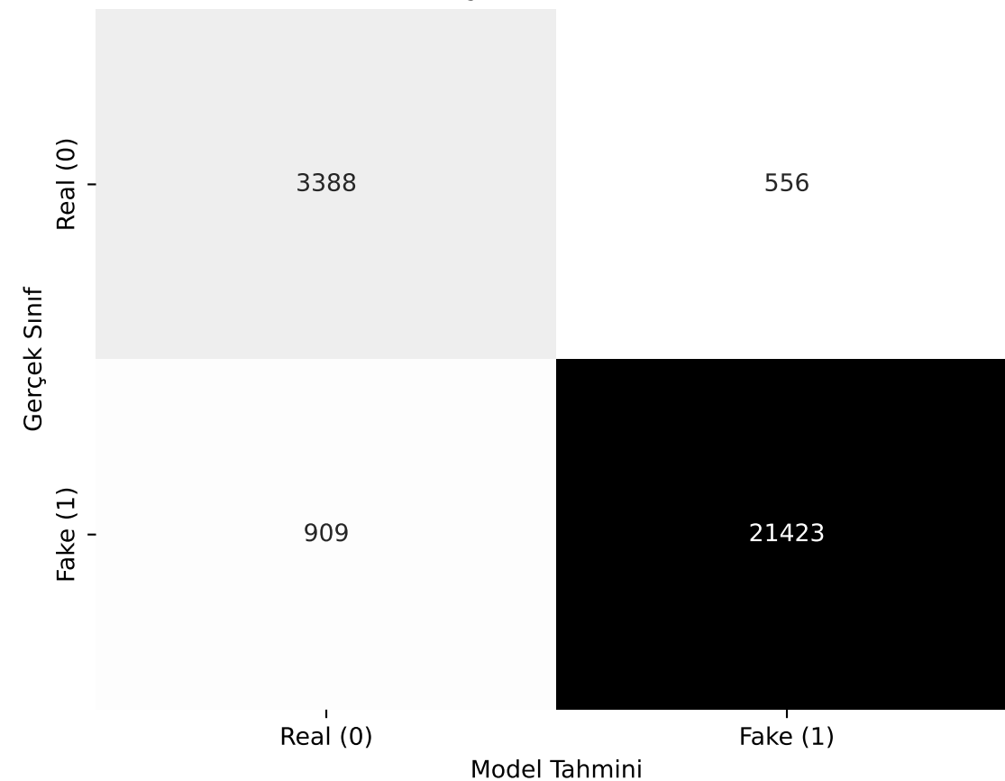
EXP005: Karmaşıklık Matrisi (EfficientNet)
