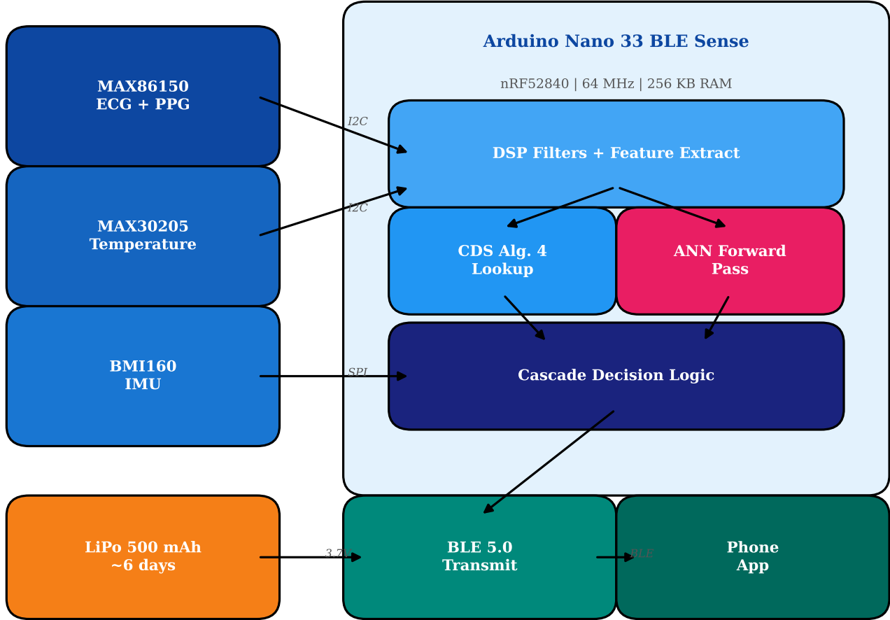
Track A: Embedded (ARM Cortex-M4F)
