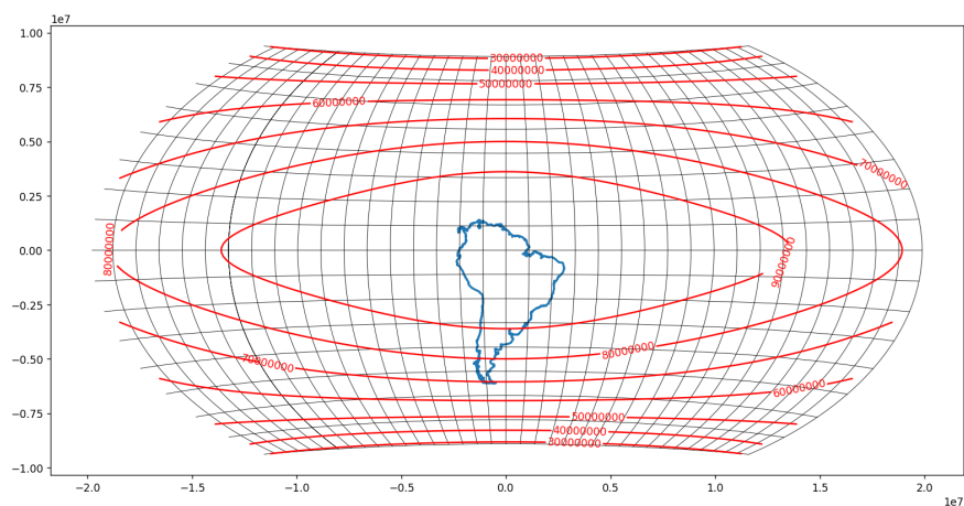
Obrázek 4: Winkel-Tripel
