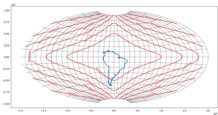
Obrázek 5: Hammer-Aitoffovo zobrazení
