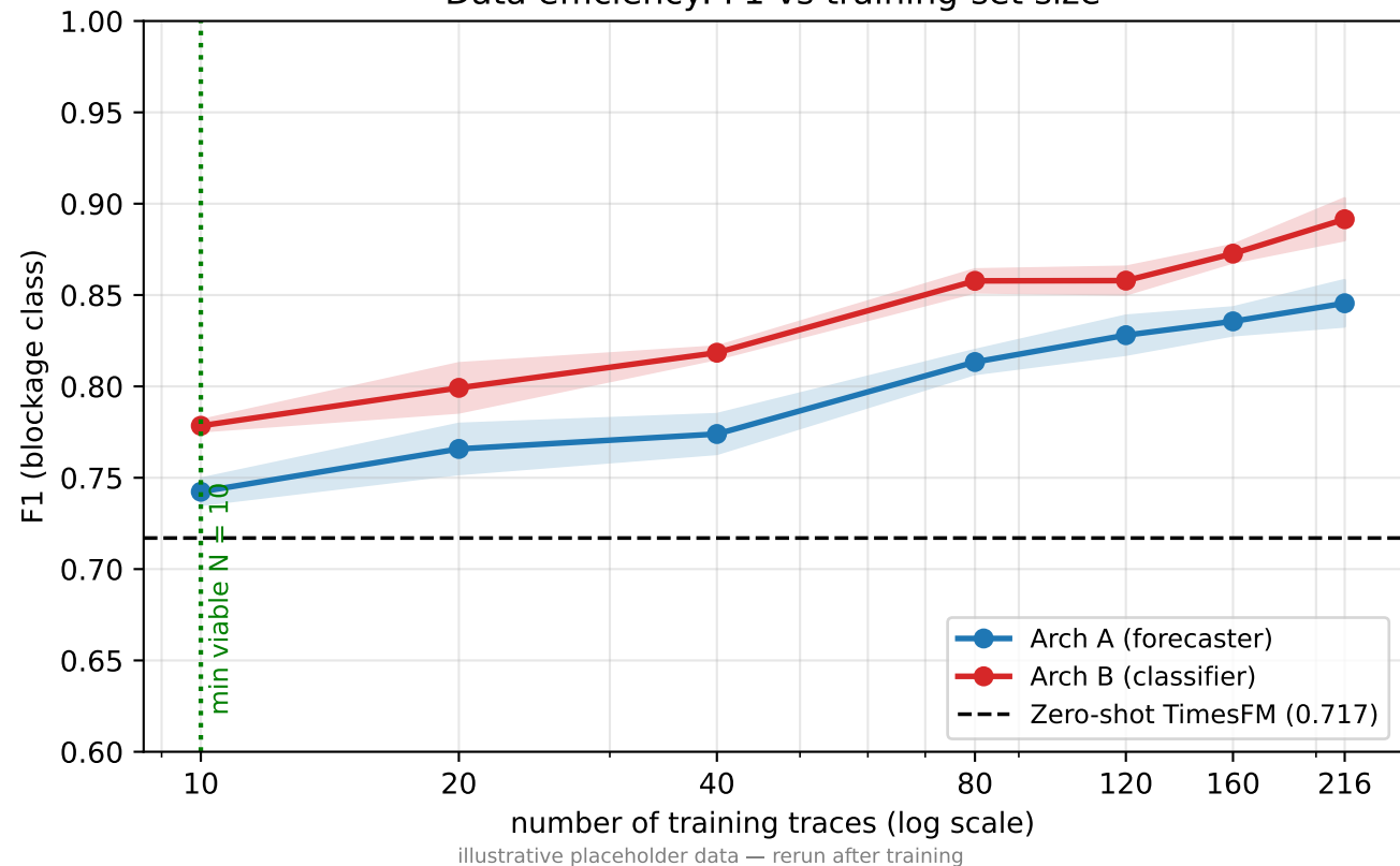
Data efficiency: F1 vs training-set size
