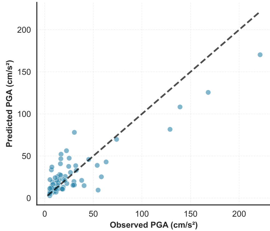
(d) Gradient Boosting Maximum PGA R^2=0.714 , RMSE=27.56
