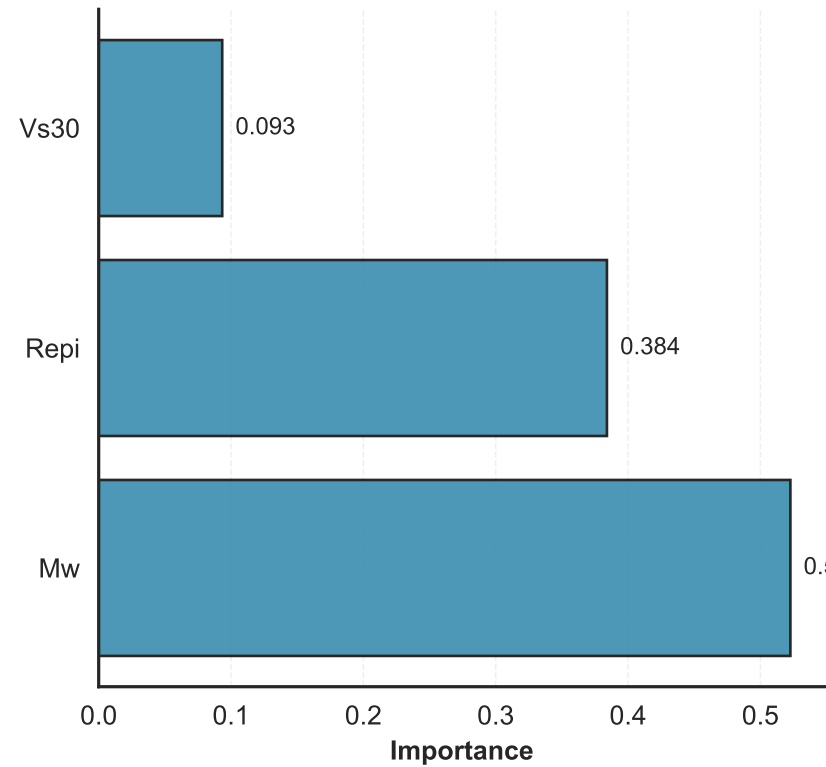
(d) Gradient Boosting Maximum PGA
