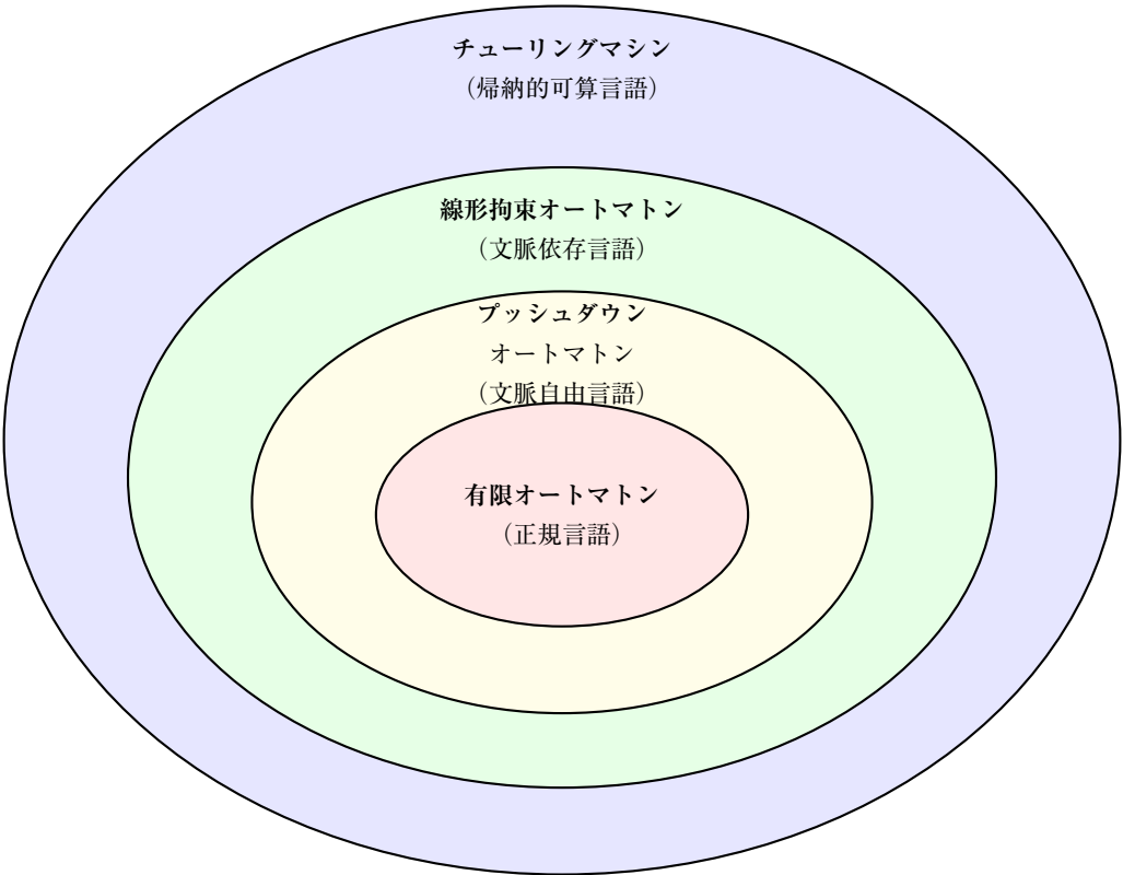
図 6.1 オートマトンの階層と言語クラスの対応 (各内側の集合は外側の集合に含まれる)
