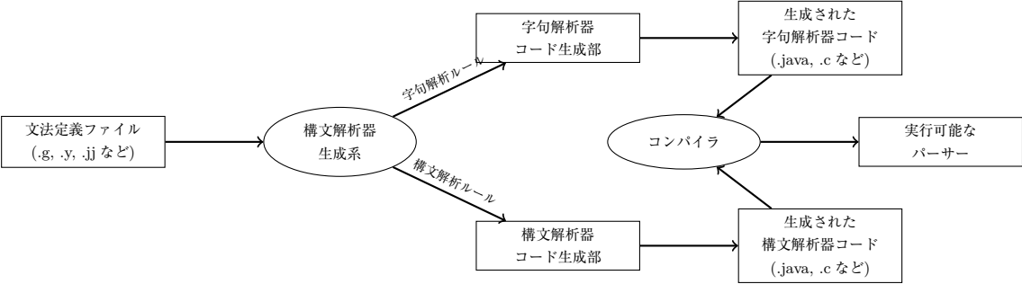
図 5.1 一般的な構文解析器生成系の処理フロー
