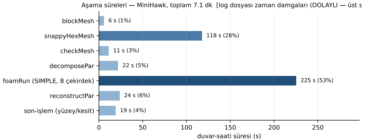
Şekil 10: Aşama süreleri (MiniHawk, 454k hücre, 8 çekirdek). Çözücü ve mesh adaptasyonu toplamın büyük kısmını alır; V&V ve rapor katmanı ölçülebilir bir ek maliyet getirmez. Yöntem figürün başlığında yazılıdır; arşivdeki bu koşu telemetri eklenmeden önce yapıldığı için dolaylı yöntemle çizilmiştir.
