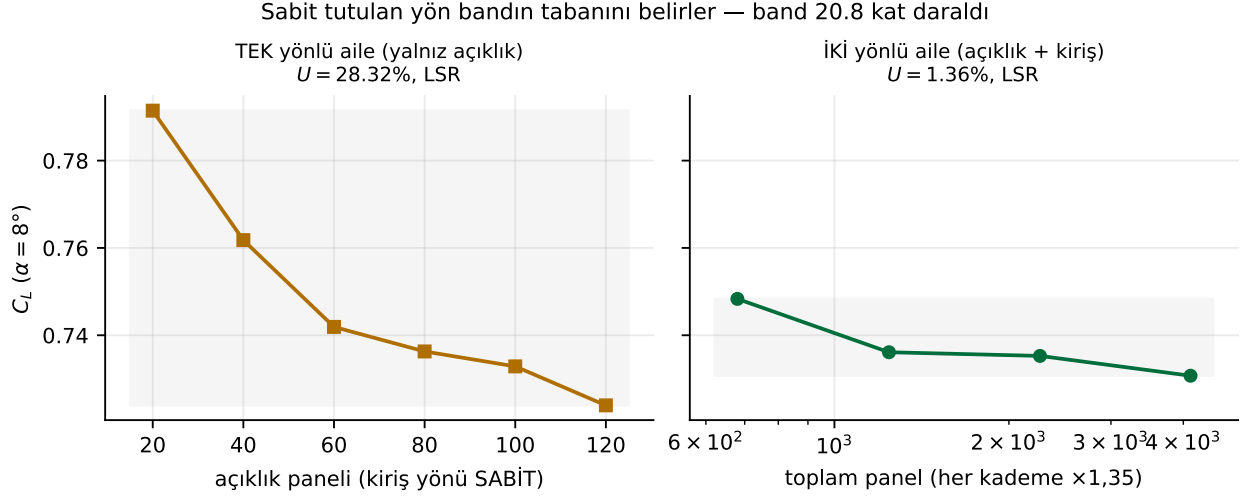
Şekil 5: Sabit tutulan yön bandın tabanını belirler. Sol: yalnız açıklık inceltirilmiş aile, asimptotik-altı ( p < 0,5 ), U = \%28,32 . Sağ: iki yön birlikte \times 1,35 inceltirilmiş aile, monoton ve süper-yakınsak ( p > 2,1 ), U = \%1,36 . Veri: vlm_iki_yonlu_yakinsama.json.
