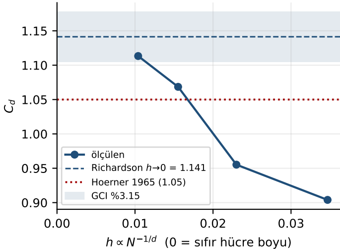
Küp — 3B araç hattı p = 2.386 , asimptotik oran 0.960
