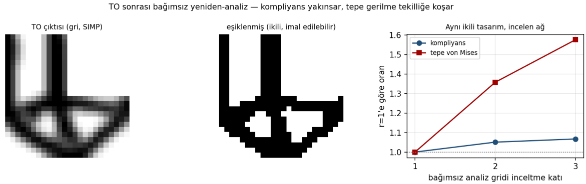
Şekil 13: TO çıktısı (gri), eşiklenmiş imal edilebilir tasarım (ikili) ve aynı ikili tasarımın incelen bağımsız ağdaki tepkisi. Kompliyan yakınsar; tepe gerilme tekilliğe koşar. Veri: topopt_bağımsız_dogrulama.json .
