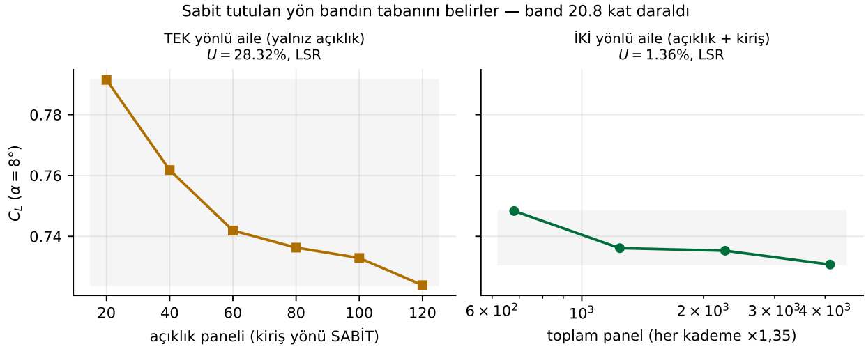
Şekil 9: Sabit tutulan yön bandın tabanını belirler. Sol: yalnız açıklık inceltilmiş aile, asimptotik-altı ( p < 0,5 ), U = \%28,32 . Sağ: iki yön birlikte \times 1,35 inceltilmiş aile, monoton ve süper-yakınsak ( p > 2,1 ), U = \%1,36 . Veri: vlm_iki_yonlu_yakinsama.json.
