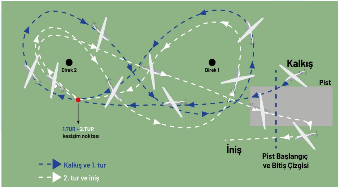
Şekil 2. Uluslararası İHA Yarışması Sabit Kanat Kategorisi Birinci Görev Uçuş Güzergâhı
