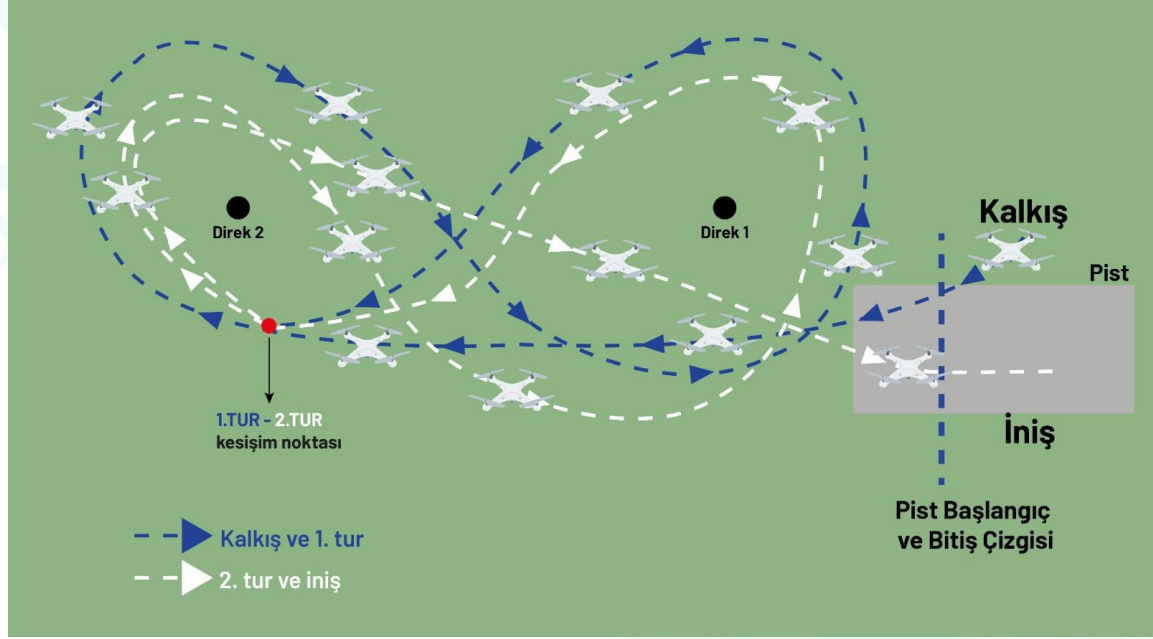
Şekil 8. Liseler Arası İHA Yarışması Döner Kanat Kategorisi Birinci Görev Uçuş Güzergâhı
