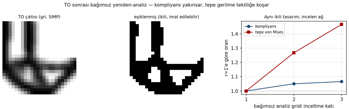
Şekil 8: TO çıktısı (gri), eşiklenmiş imal edilebilir tasarım (ikili) ve aynı ikili tasarımın incelen bağımsız ağdaki tepkisi. Kompiyans yakınsar; tepe gerilme tekilliğe koşar. Veri: topopt_bagimsiz_dogrulama.json.
