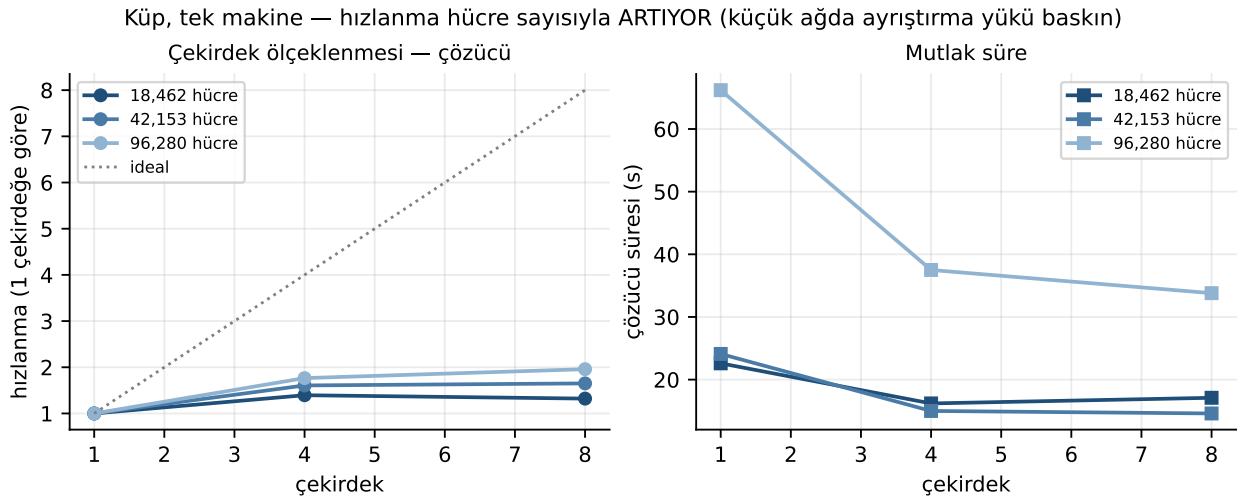
Şekil 11: Çekirdek ölçeklenmesi ve mutlak süre. Kesikli çizgi ideal hızlanmadır; ölçülen eğriler hep altındadır. Veri: basarim_matrisi.json .
