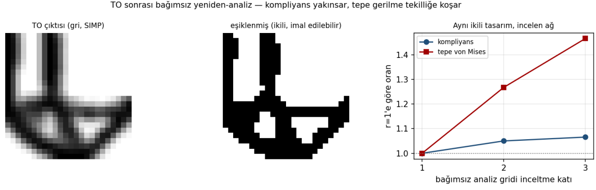
Şekil 8: TO çıktısı (gri), eşiklenmiş imal edilebilir tasarım (ikili) ve aynı ikili tasarımın incelen bağımsız ağdaki tepkisi. Kompiyans yakınsar; tepe gerilme tekilliğe koşar. Veri: toptopt_bagimsiz_dogrulama.json.
