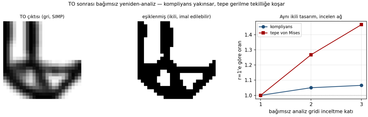
Şekil 8: TO çıktısı (gri), eşiklenmiş imal edilebilir tasarım (ikili) ve aynı ikili tasarımın incelen bağımsız ağıdaki tepkisi. Kompiyans yakınsar; tepe gerilme tekilliğe koşar. Veri: topopt_bagimsiz_dogrulama.json .
