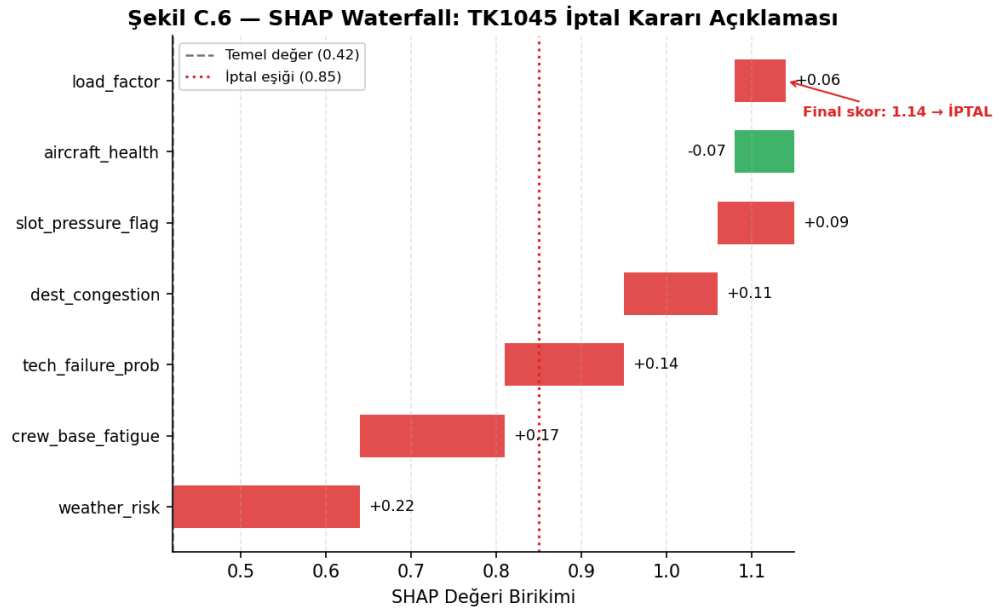
Şekil 15.3: Şekil C.6 — SHAP Waterfall
