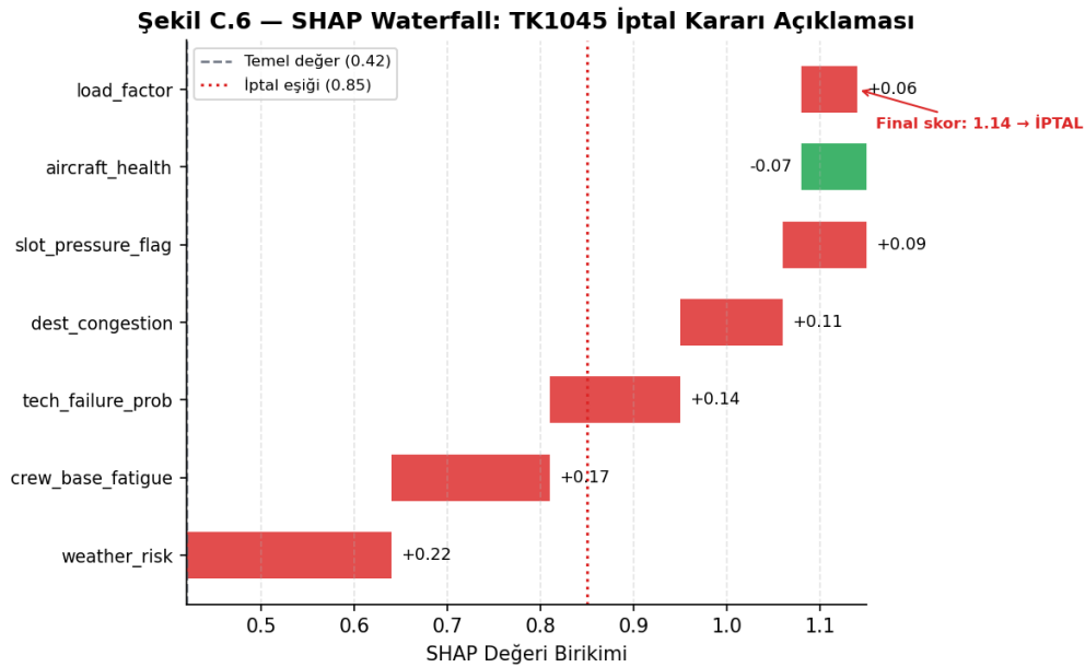
Şekil 15.1: Şekil C.6 — SHAP Waterfall
