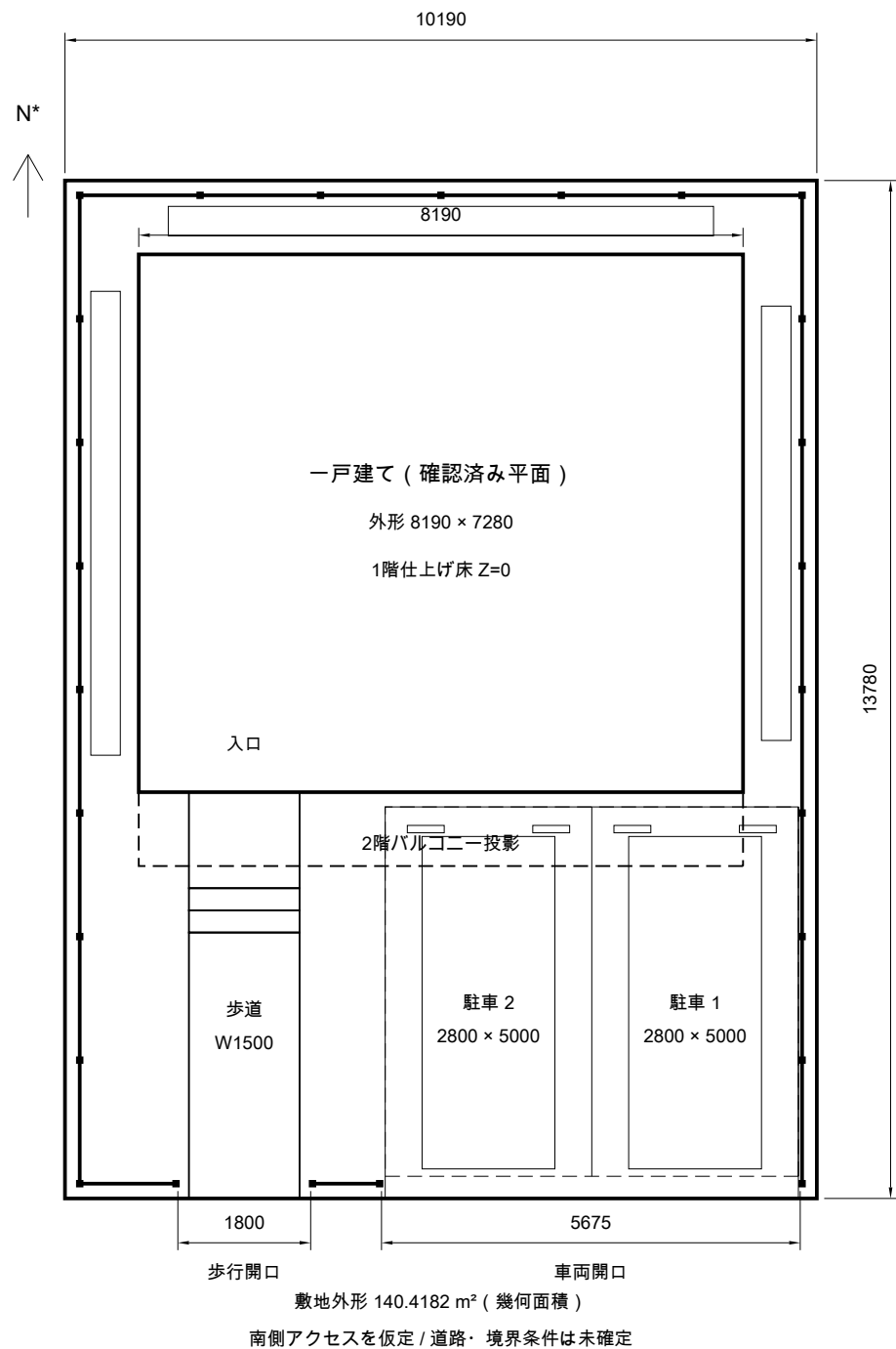
01 配置図
