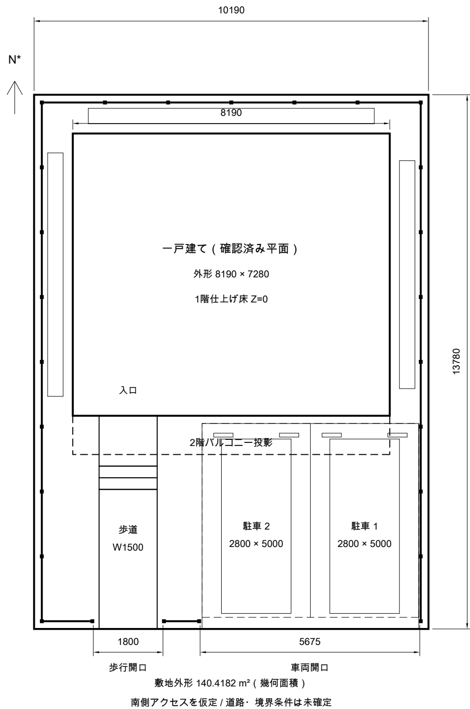
01 配置図
