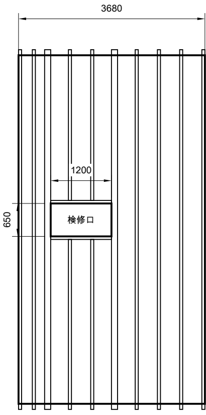
02 小屋裏床組・ 検修口 / 1:75
