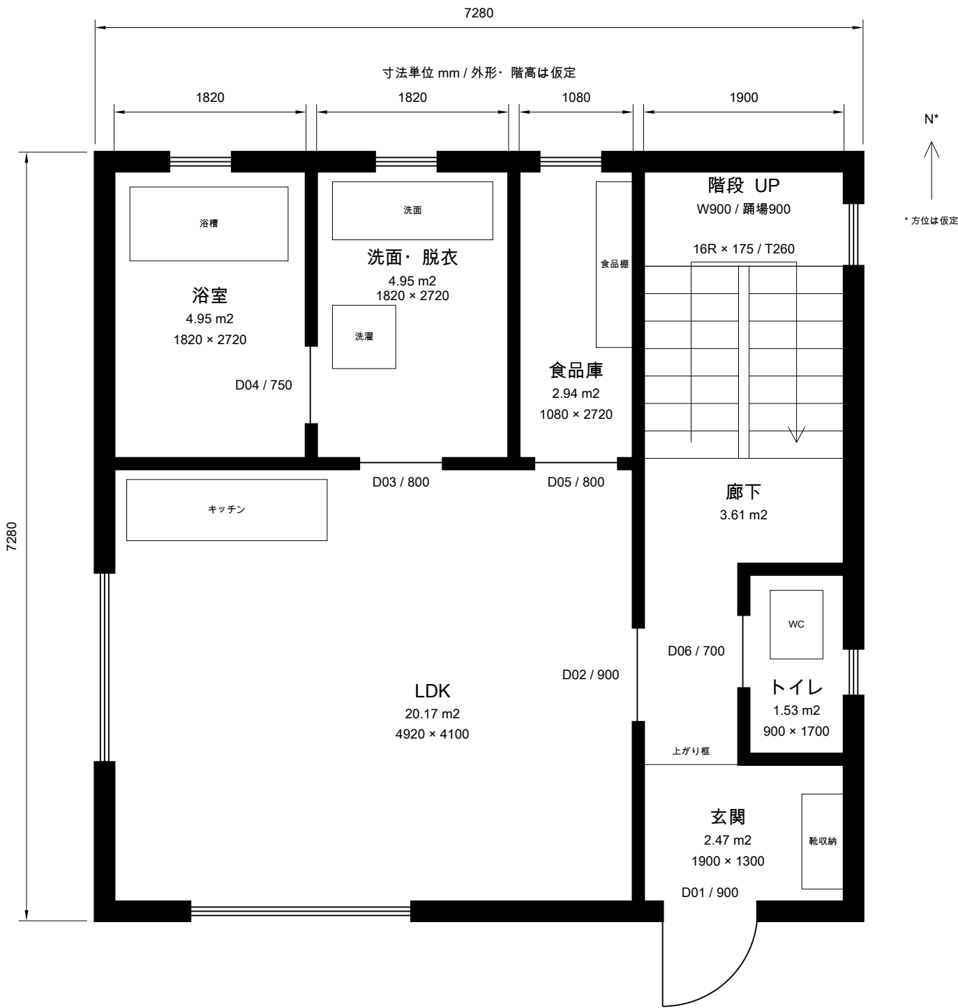
R02 / 1階 平面図 ( 参考計画 )
