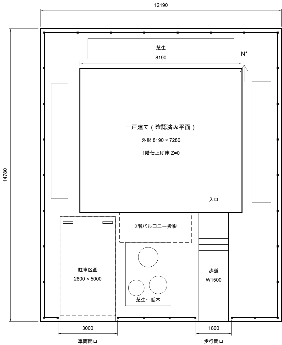
01 配置図
