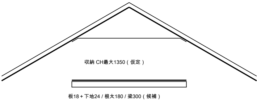
03 東西参考断面 / 1:75 ( Zは実座標 )
