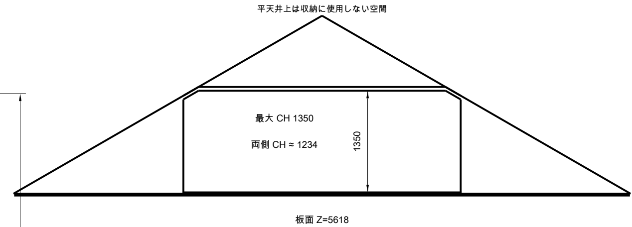
参考断面 ( 東西・ Y=2000 ) / 屋根外形維持
