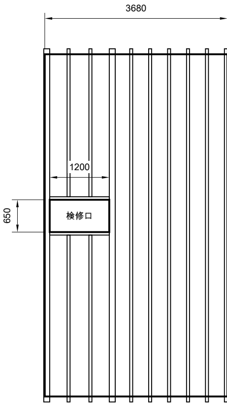
02 小屋裏床組・ 検修口 / 1:75
