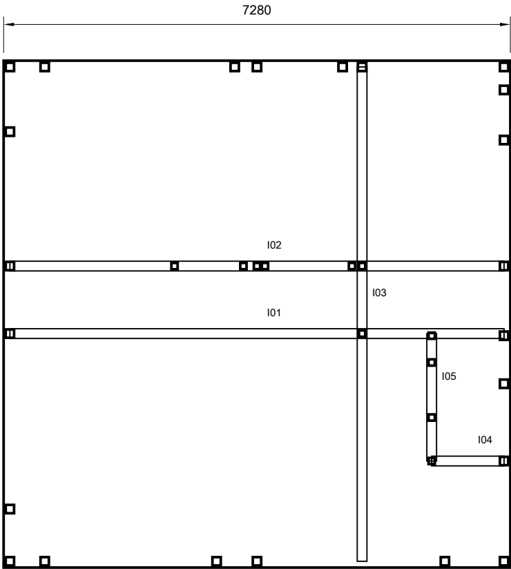
01 基礎支持線候補 / 1:75
