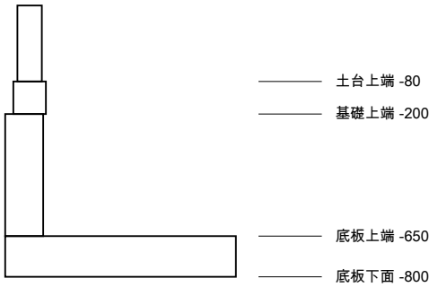
04 基礎参考断面 / 1:25
