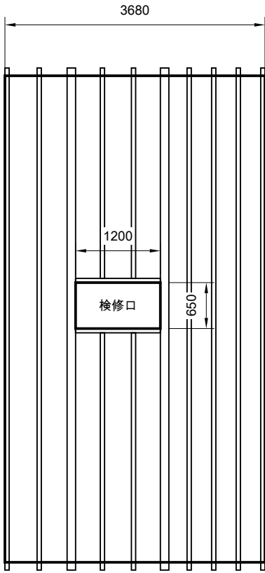
02 小屋裏床組・ 検修口 / 1:75
