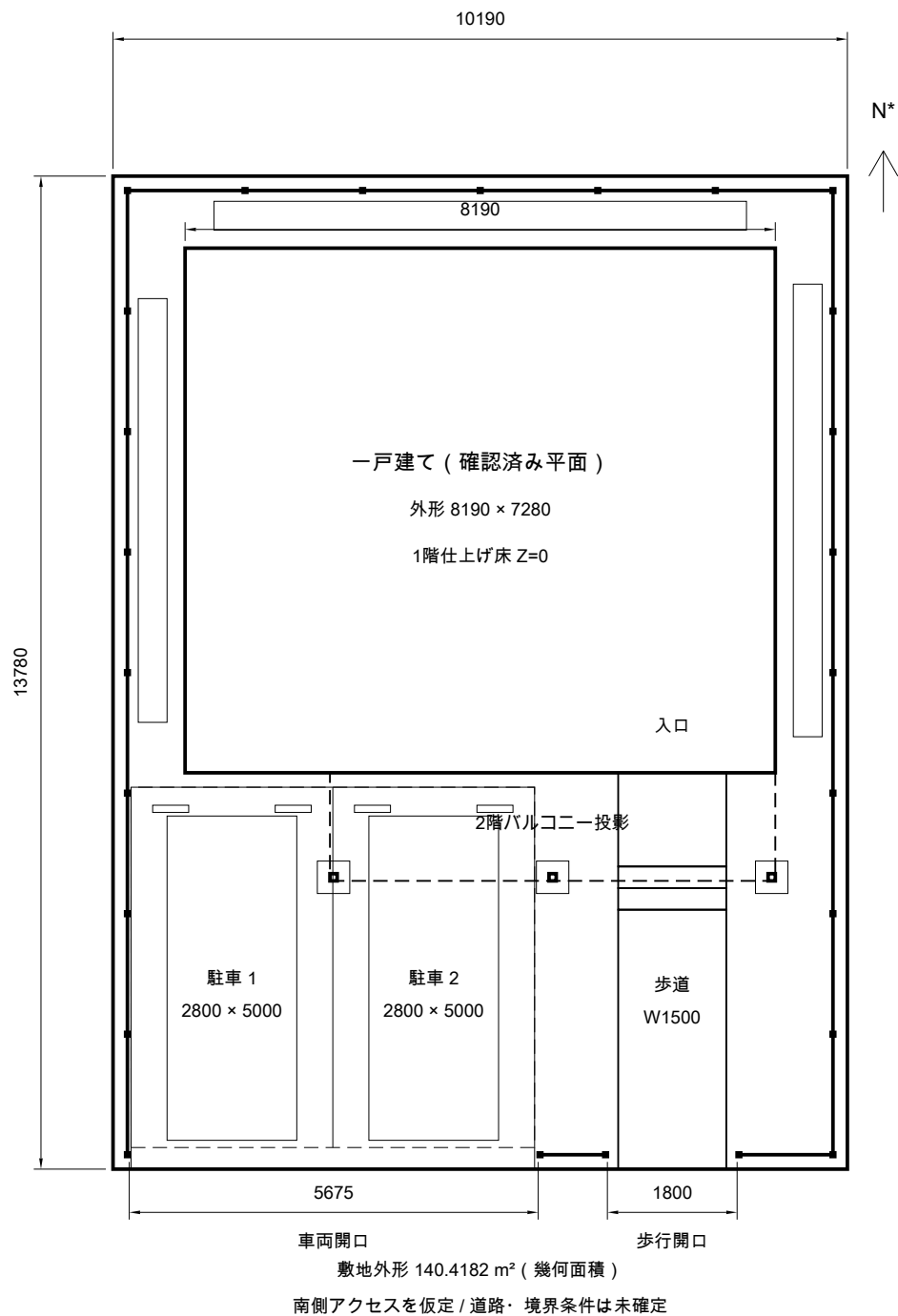
01 配置図
