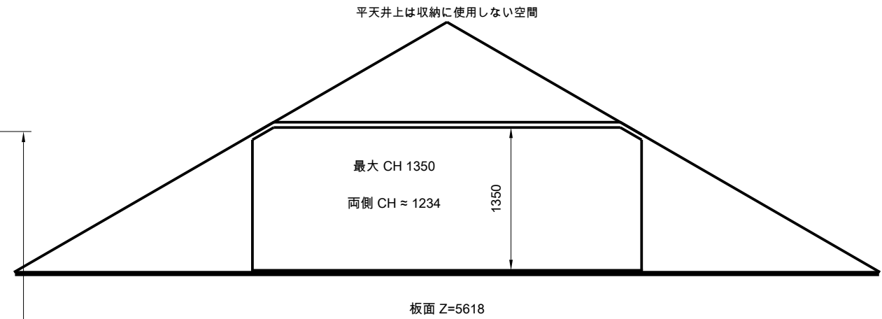
参考断面 (東西・ Y=2000) / 屋根外形維持
