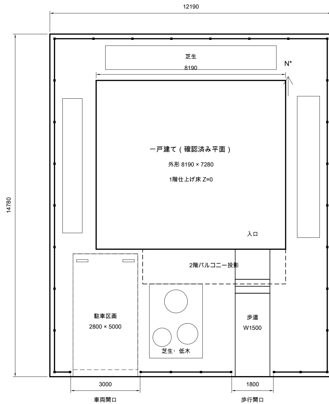
01 配置図
