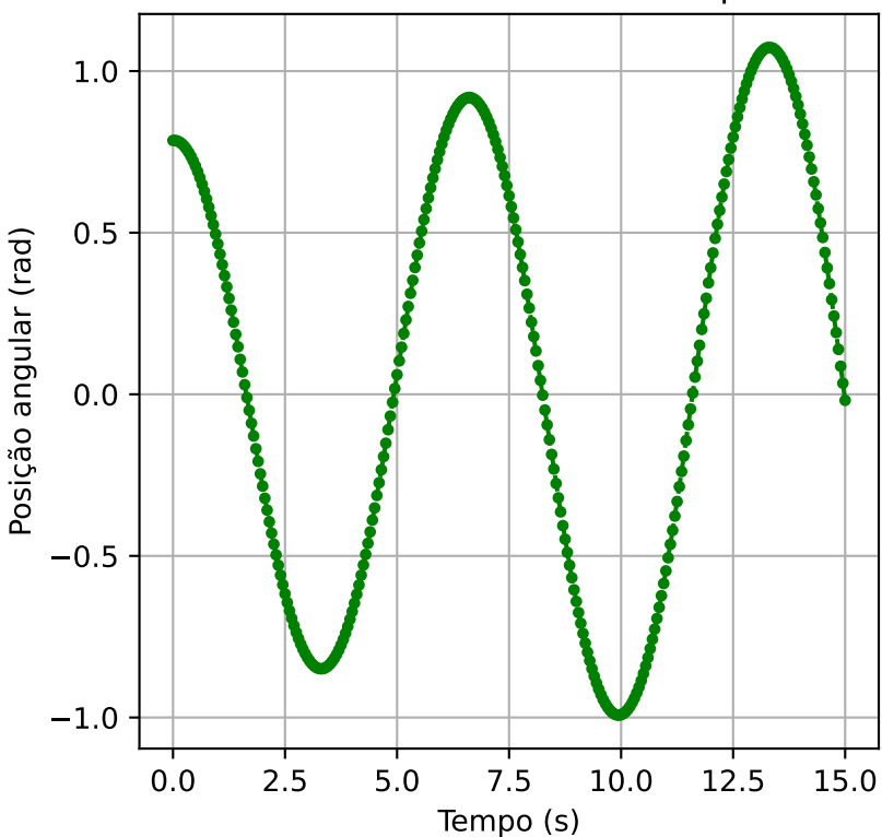
Resultado numérico - Runge-Kutta clássico
