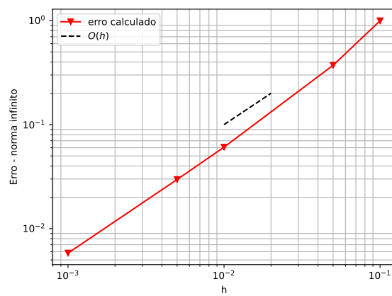
Figura 2: Erro do método Euler Explícito
