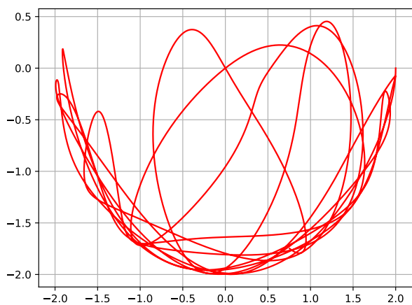
(a) Trajetória, com q_1(0) = q_2(0) = \frac{\pi}{2}
