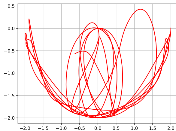
(b) Trajetória, com q_1(0) = \frac{\pi}{2} e q_2(0) = \frac{\pi}{2} + 10^{-2}
