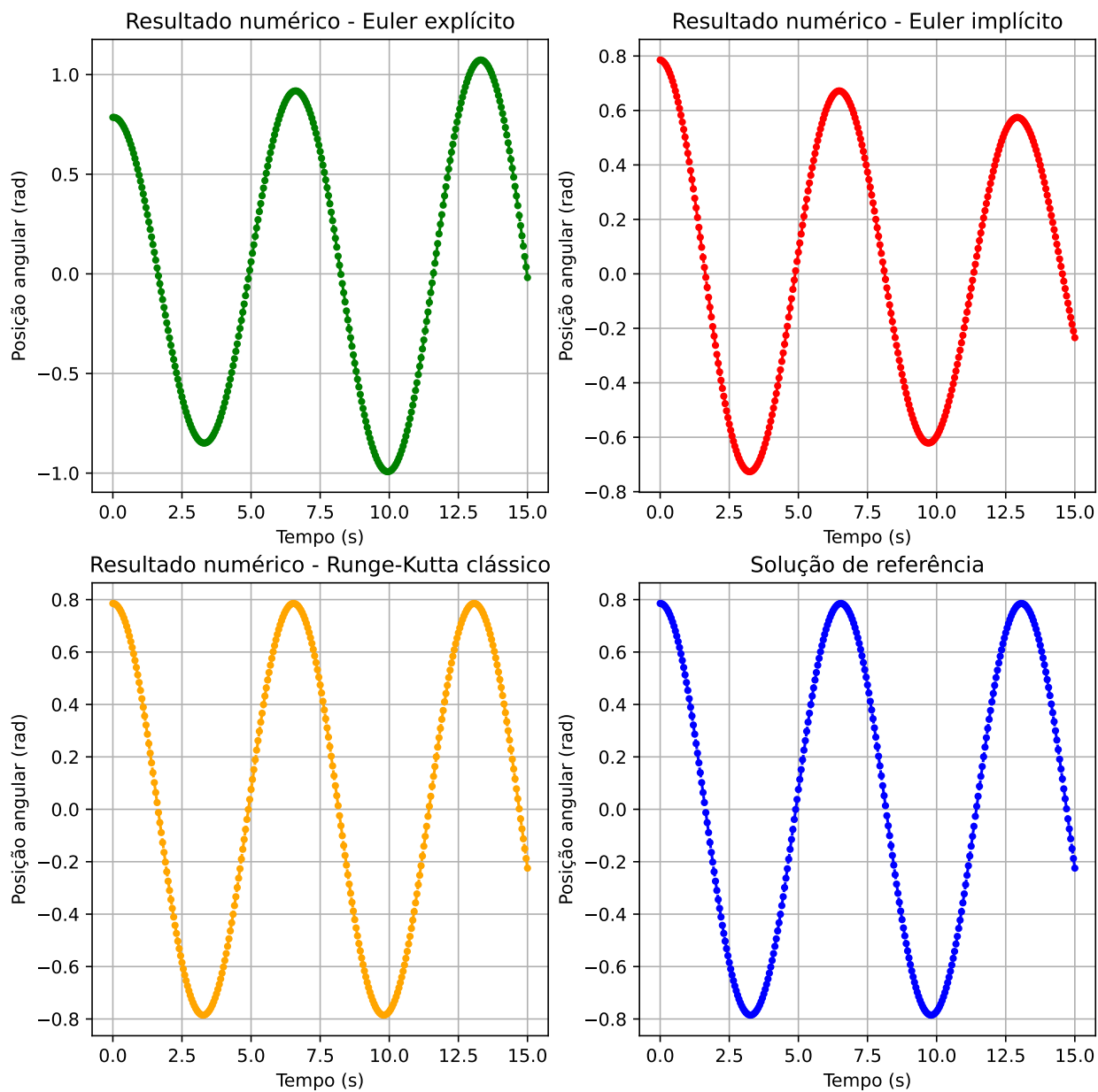
Figura 1: Posição angular em função do tempo
