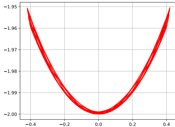
Figura 7: Experimento 1, com q_1(0) = q_2(0) = 0.2
