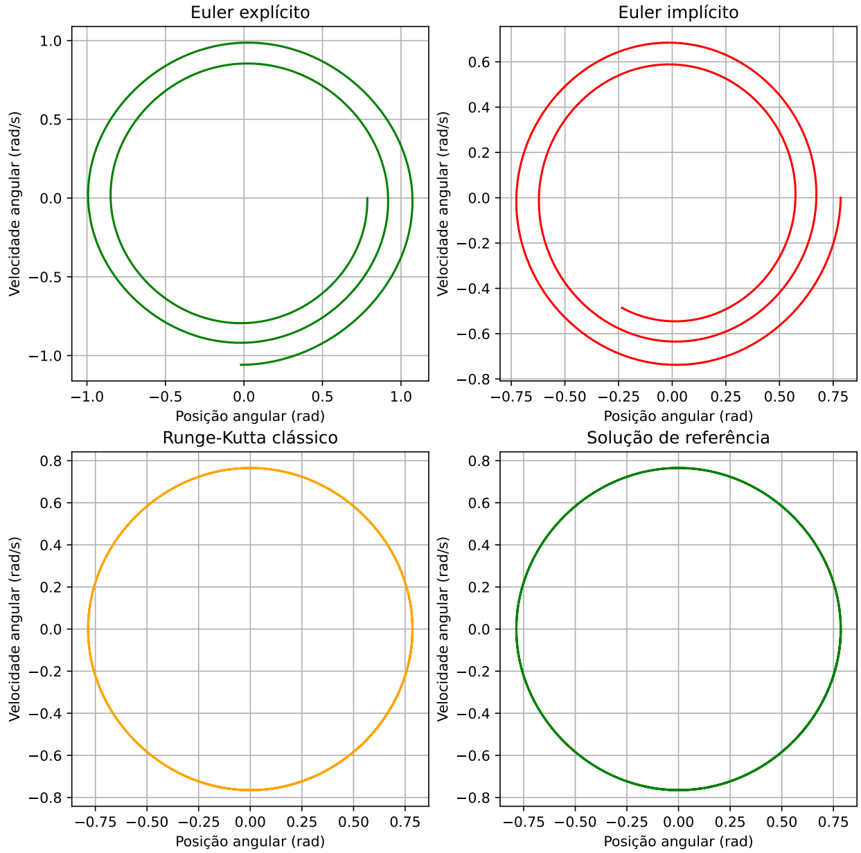
Figura 5: Velocidade angular em função da posição angular
