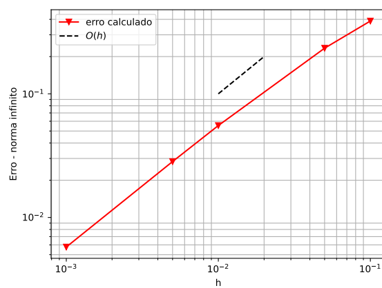
Figura 3: Erro do método Euler Implícito
