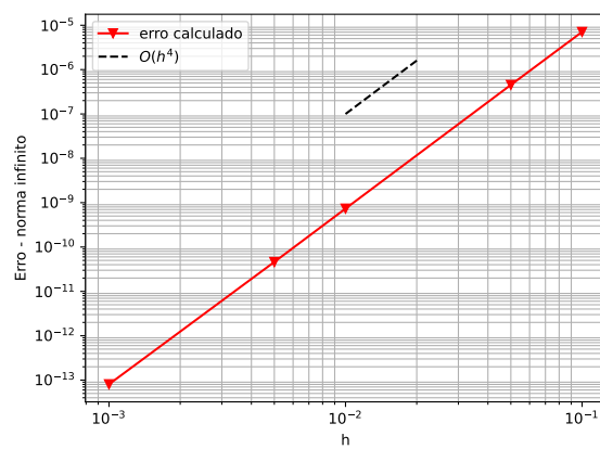
Figura 4: Erro do método RK4
