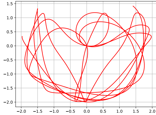
Figura 6: Trajetória de um pêndulo, com q_1(0) = q_2(0) = \frac{3\pi}{4}
