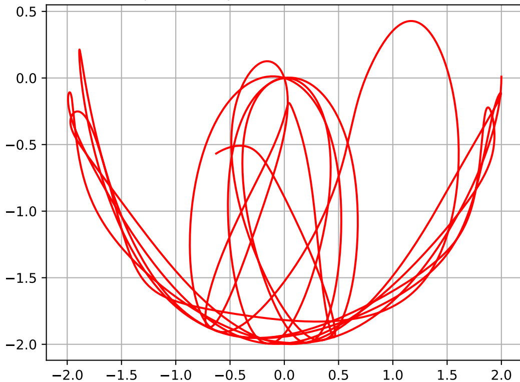
Trajetória do pêndulo - Condição inicial 2
