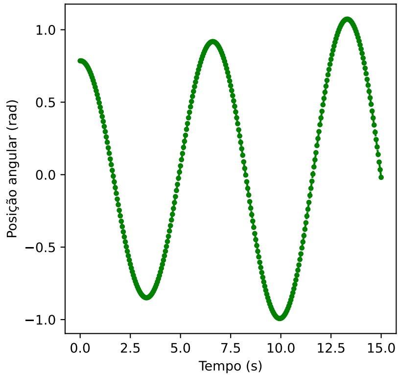
Resultado numérico - Runge-Kutta clássico
