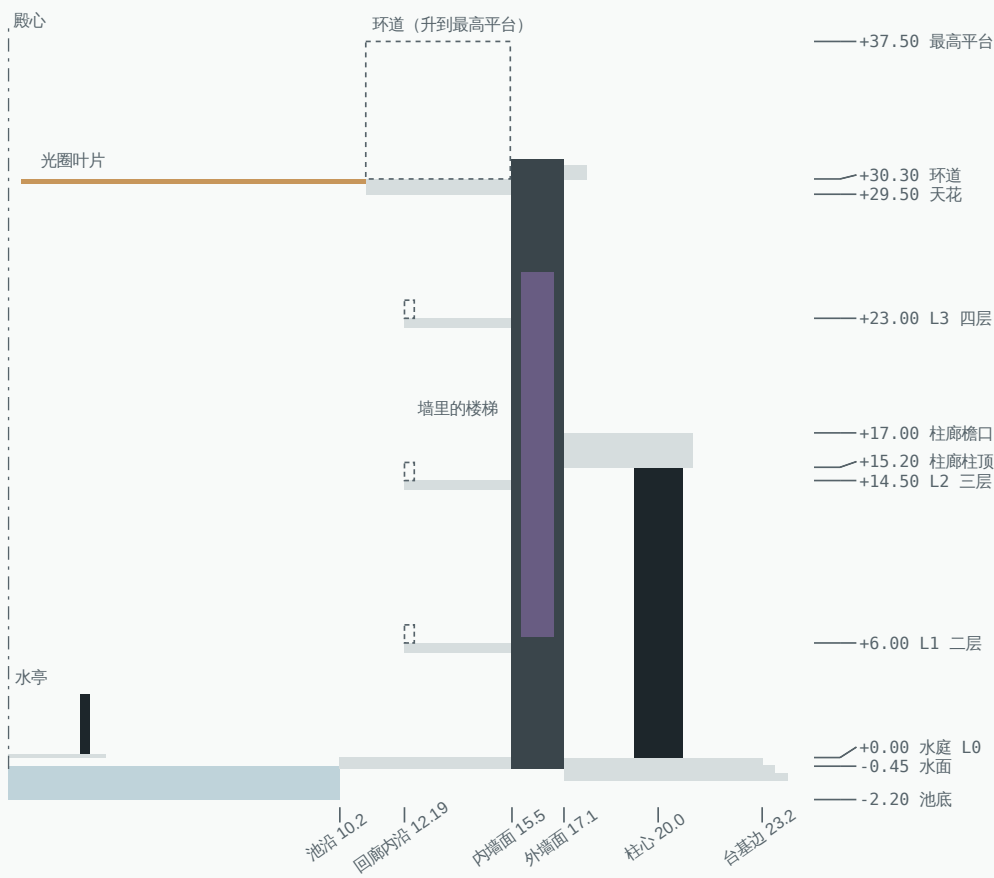
径向半剖面（左边是殿心，右边是殿外）。竖向比例是横向的 1/1.7，只看高度关系。
