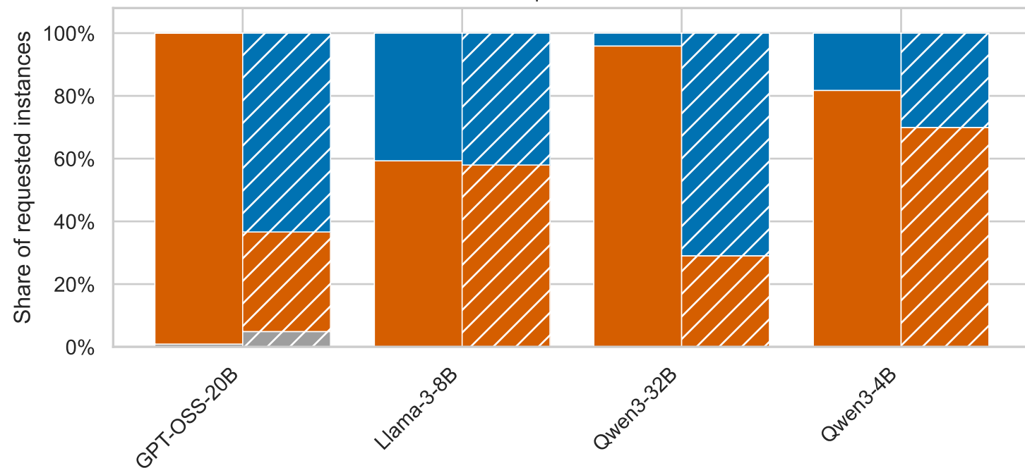
Pairwise | TREC-DL-2019
