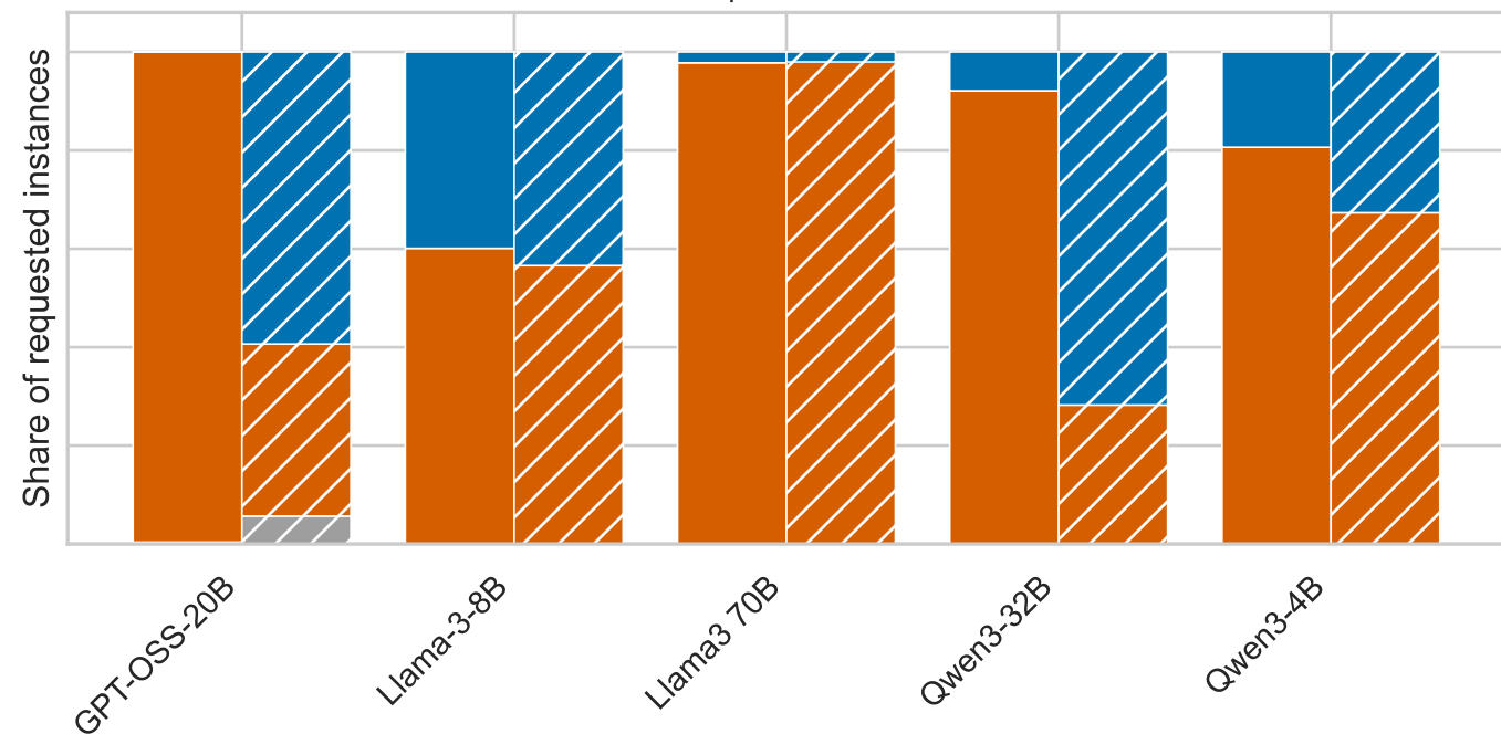
Pairwise | TREC-DL-2020
