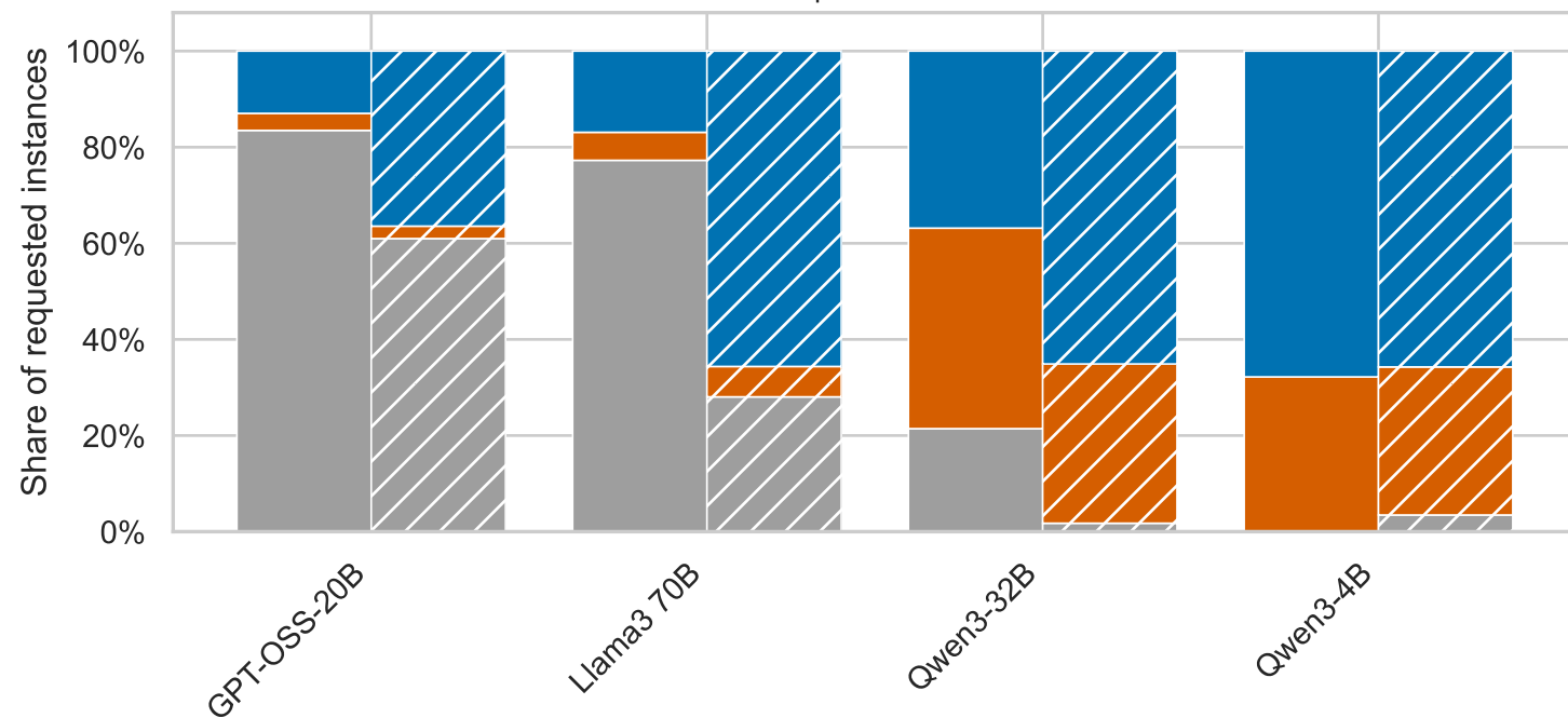
Listwise | TREC-DL-2019
