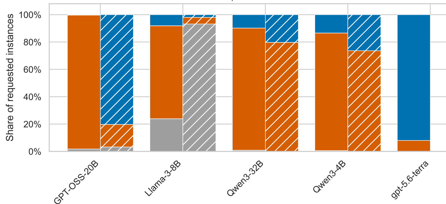
Setwise | TREC-DL-2019
