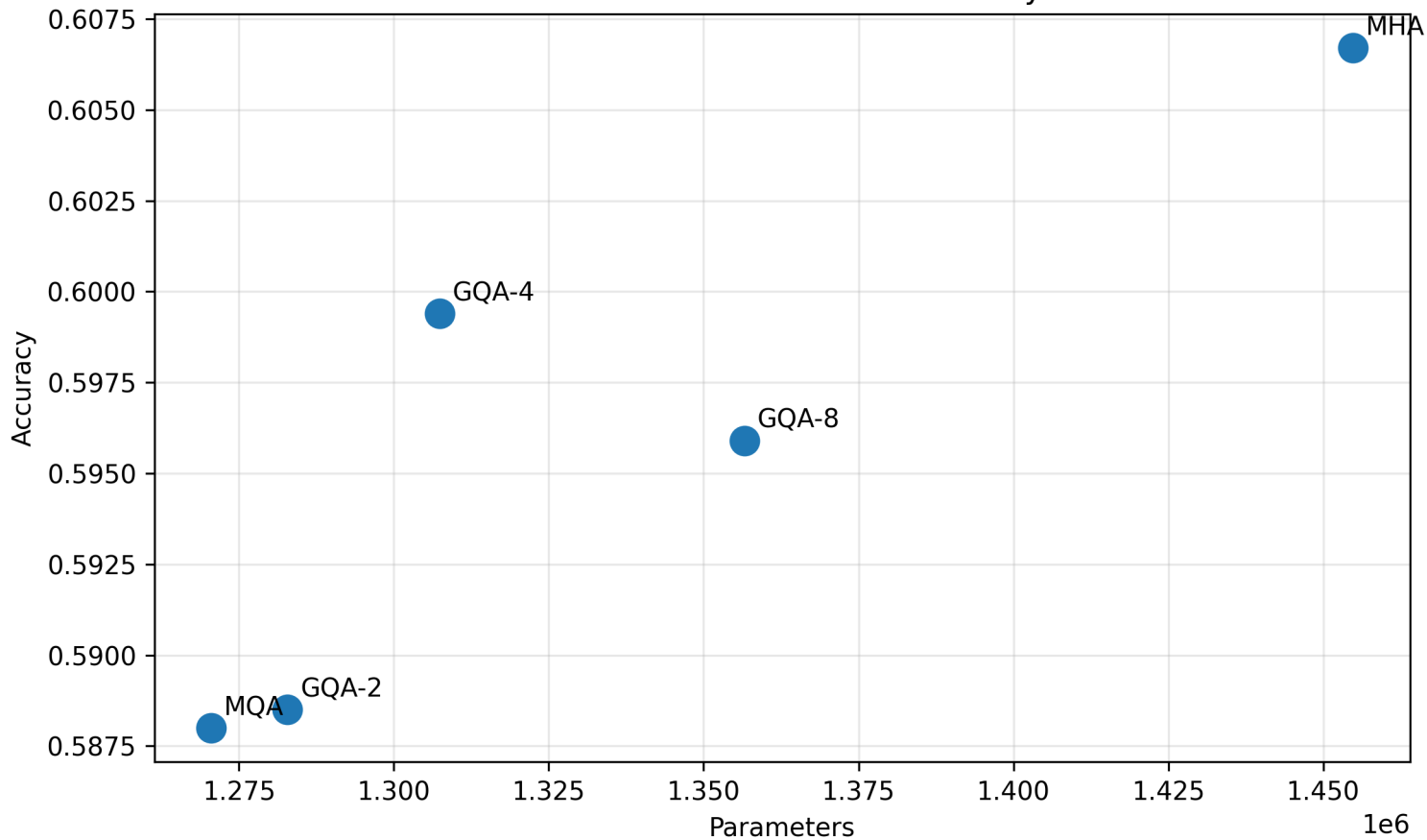
ViT: Parameter Count vs Accuracy
