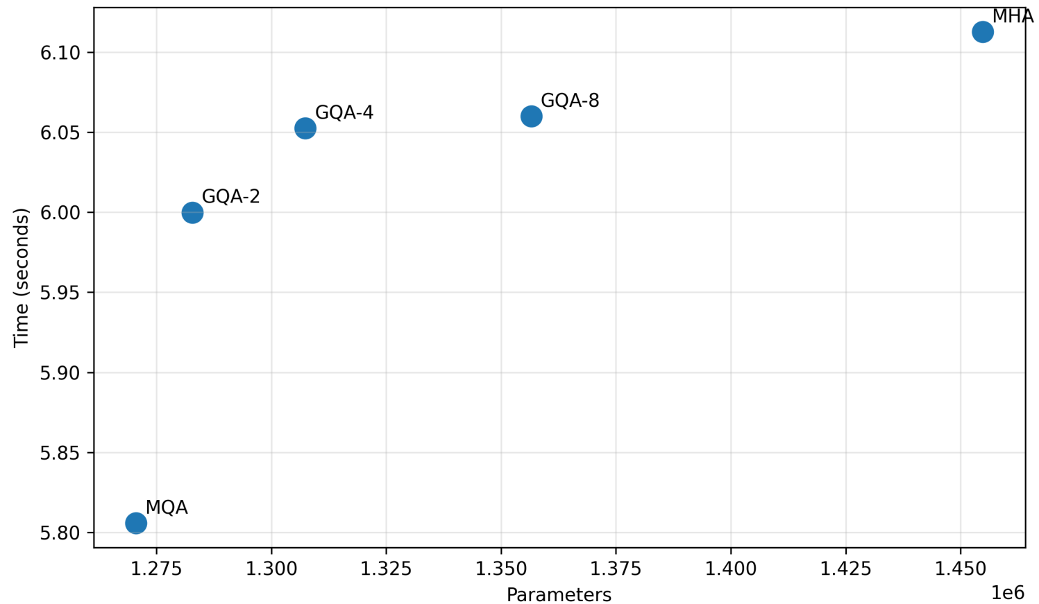
ViT: Parameter Count vs Inference Time
