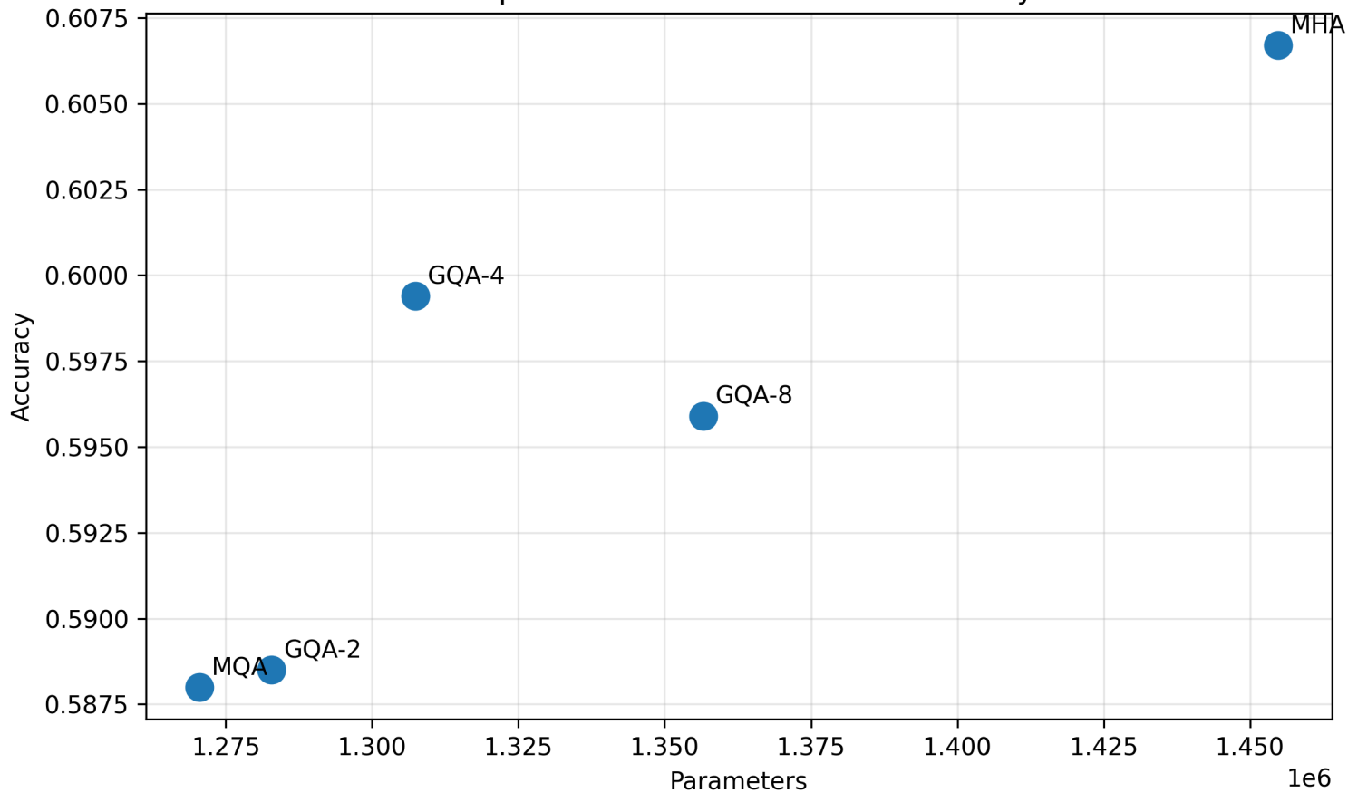
SimpleViT: Parameter Count vs Accuracy
