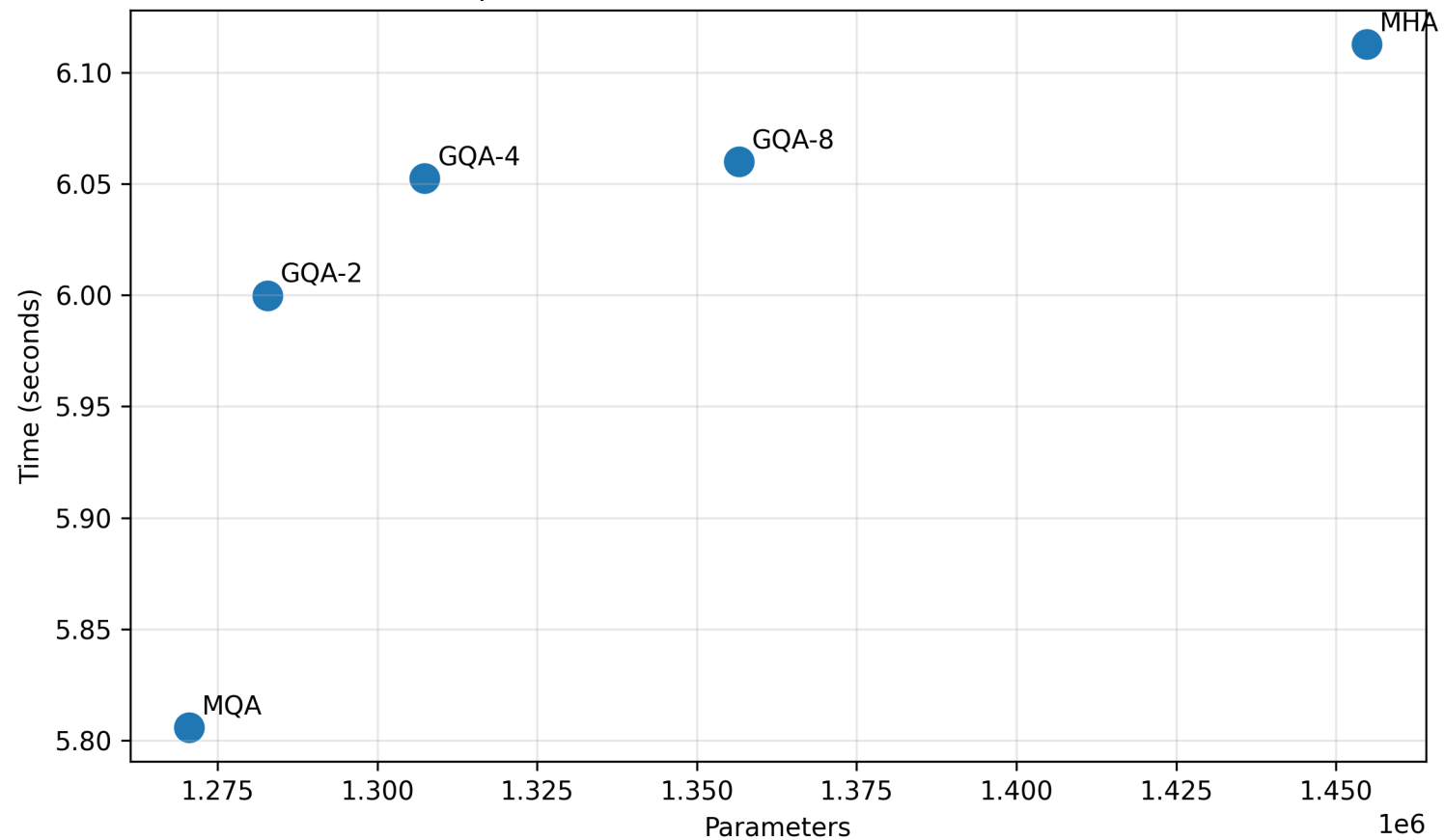
SimpleViT: Parameter Count vs Inference Time
