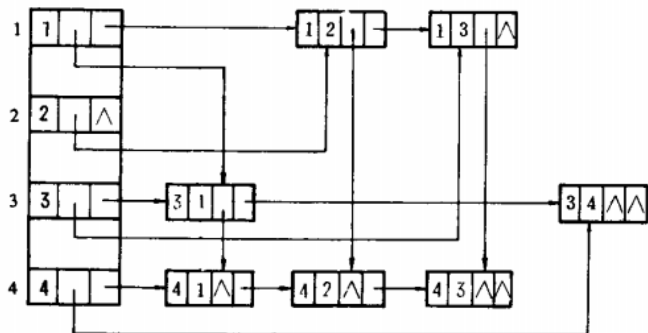
有向图的十字链表
