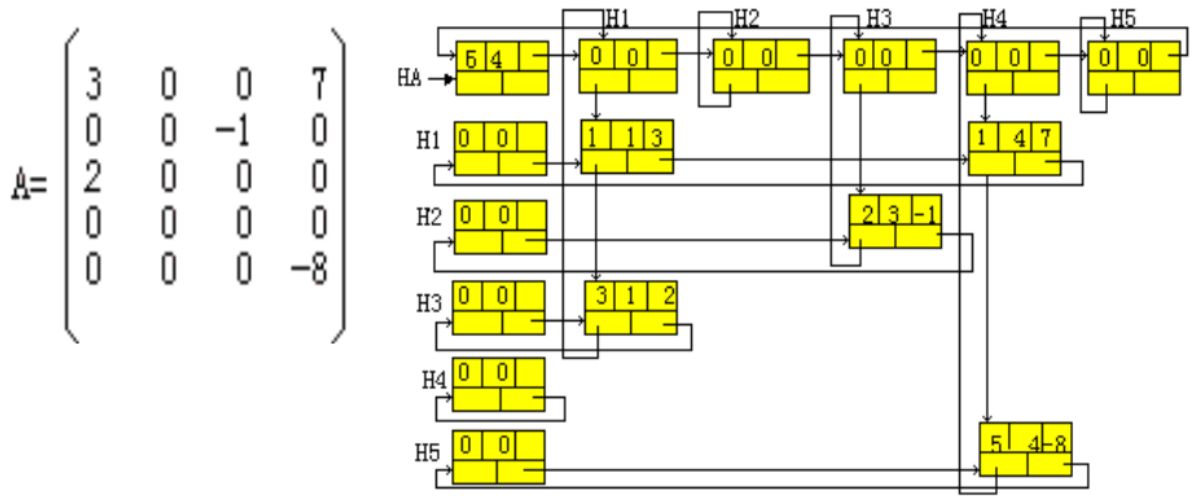
用十字链表表示的稀疏矩阵 A
