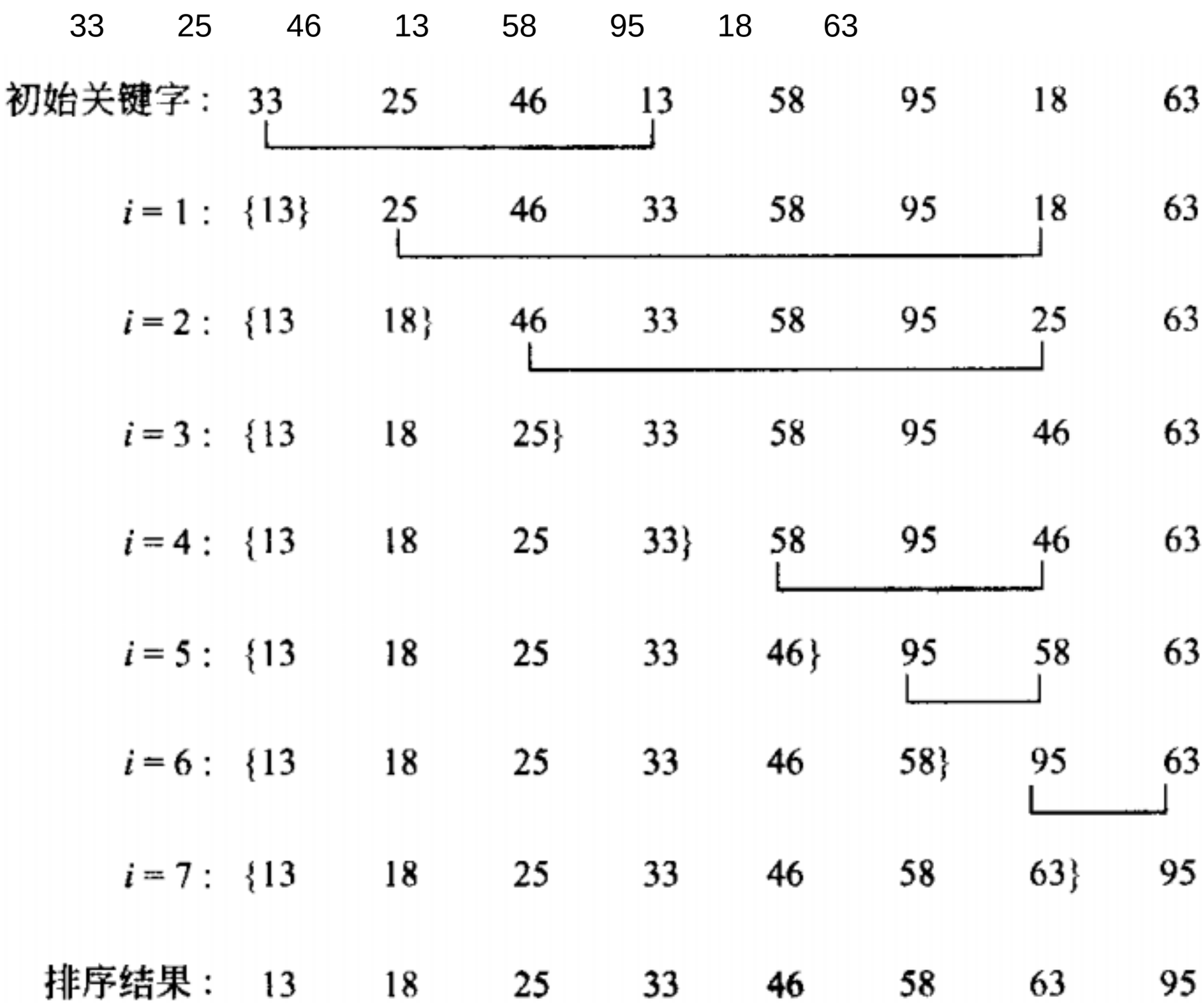
简单选择排序的过程示意图。
