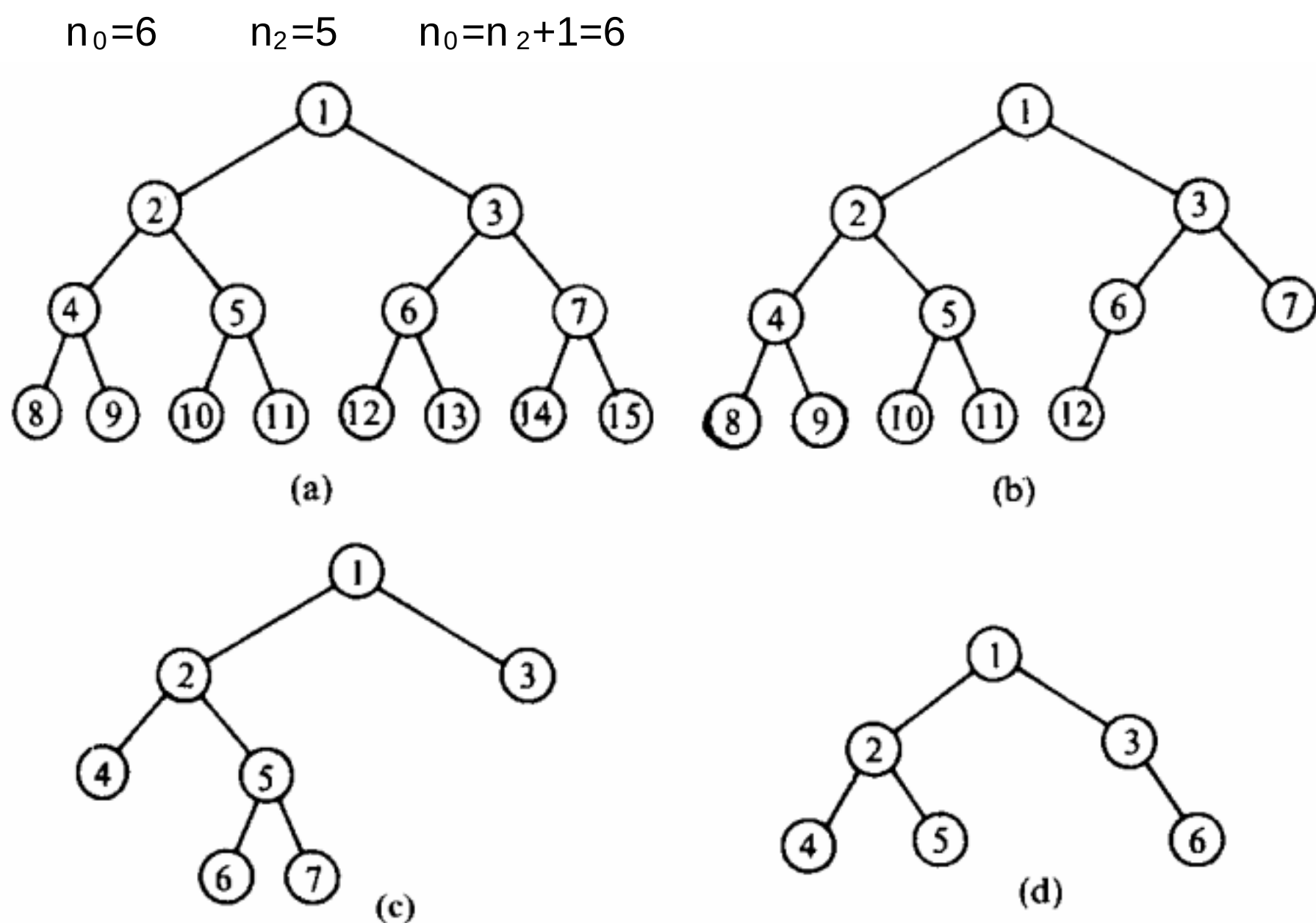
图 5.3 特殊形态的二叉树
