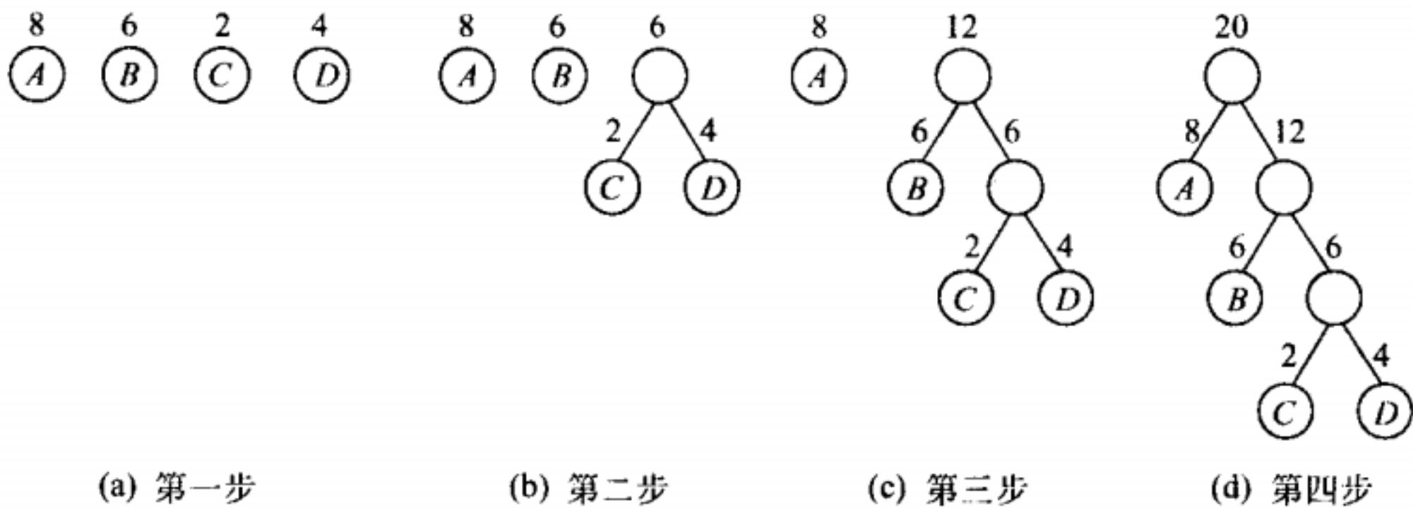
构造赫夫曼树的过程
