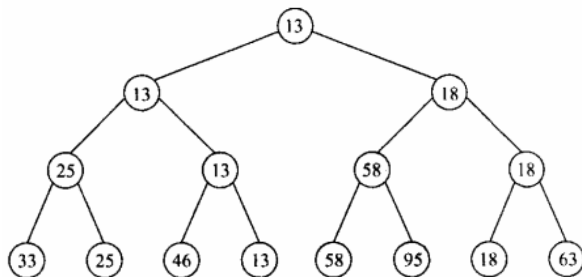
(a) 第一趟选择最小关键字过程示意
