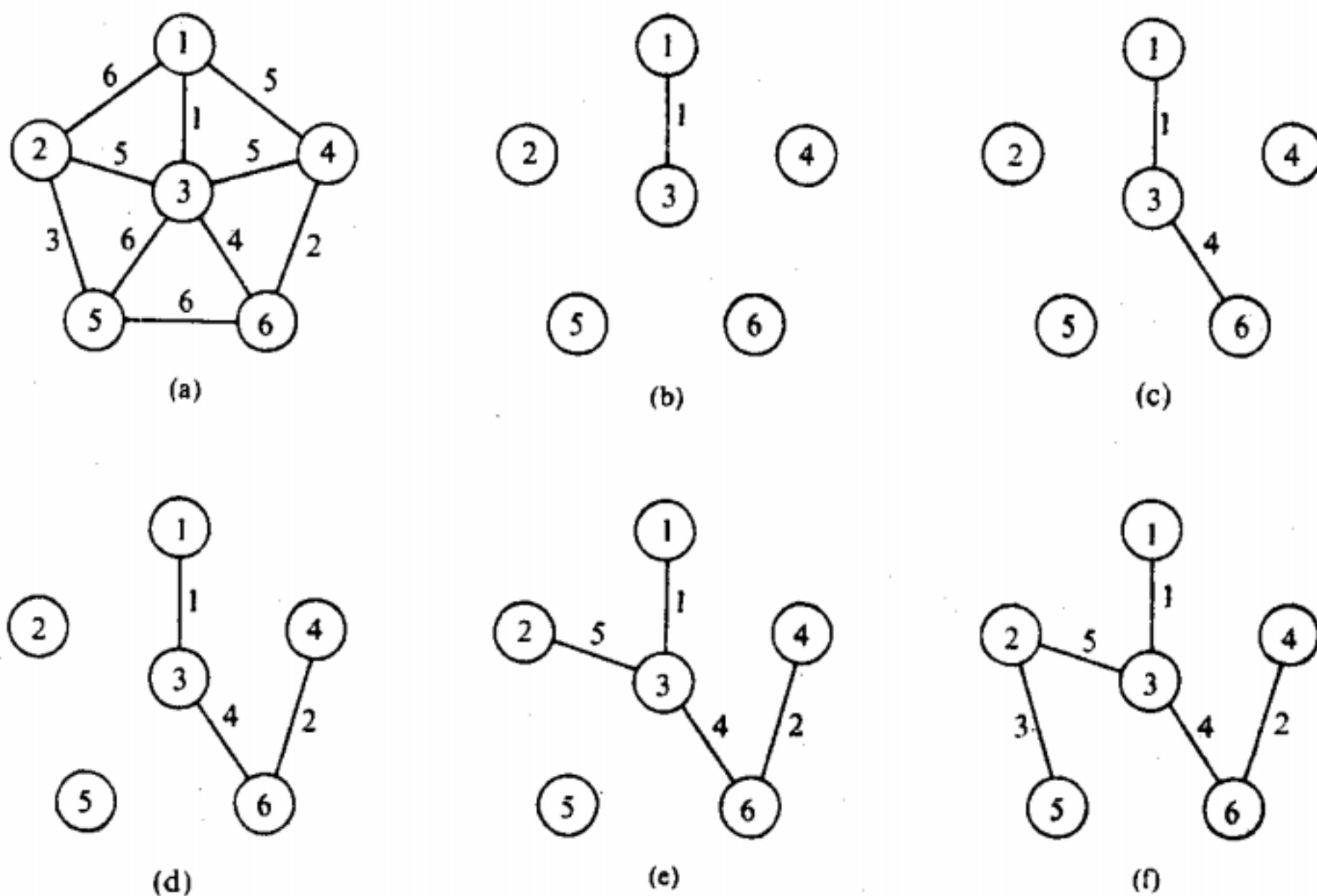
图 6.24 普里姆算法构造最小生成树的过程
