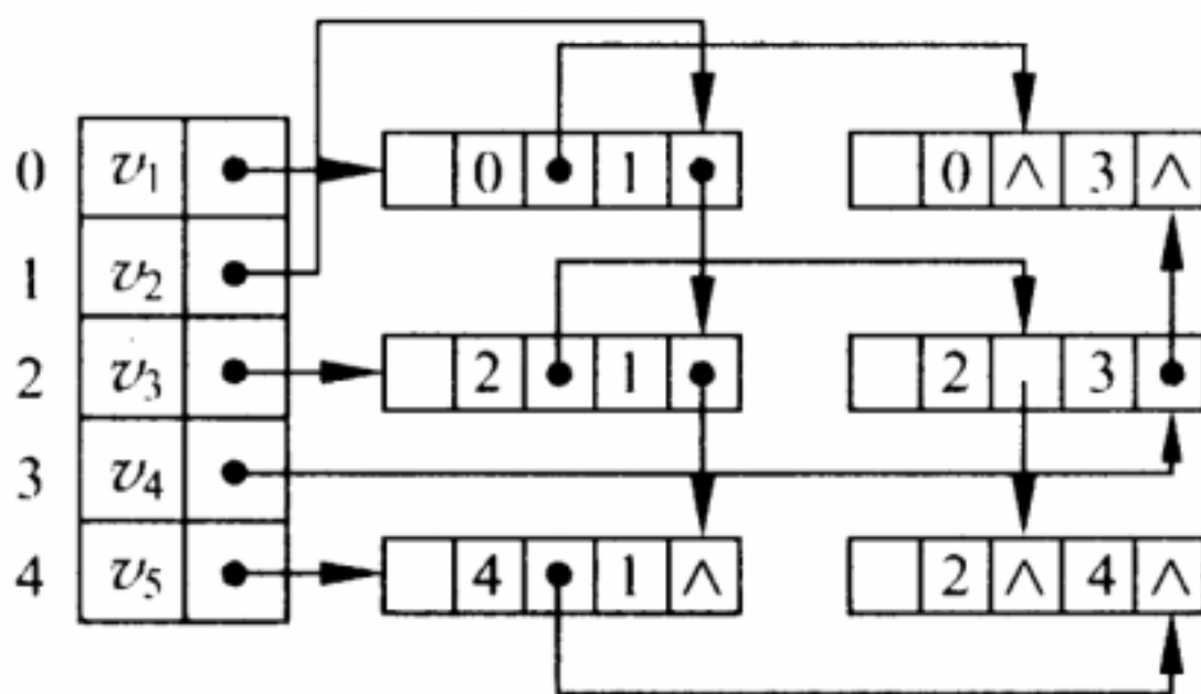
无向图 G2的邻接多重表
