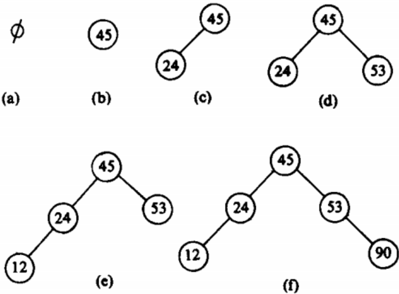
二叉排序树的构造过程
