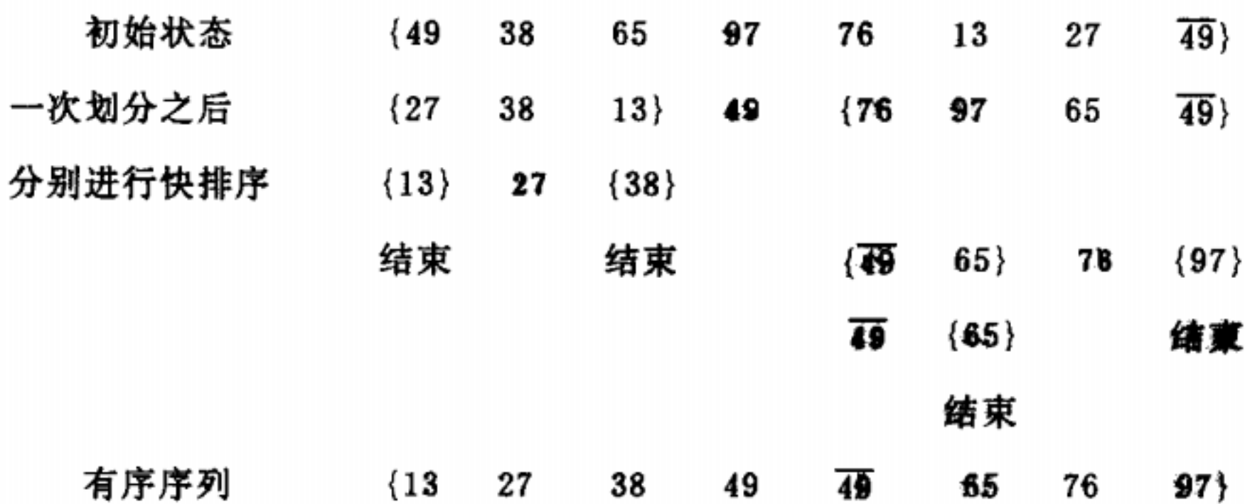
快速排序的过程示意图
