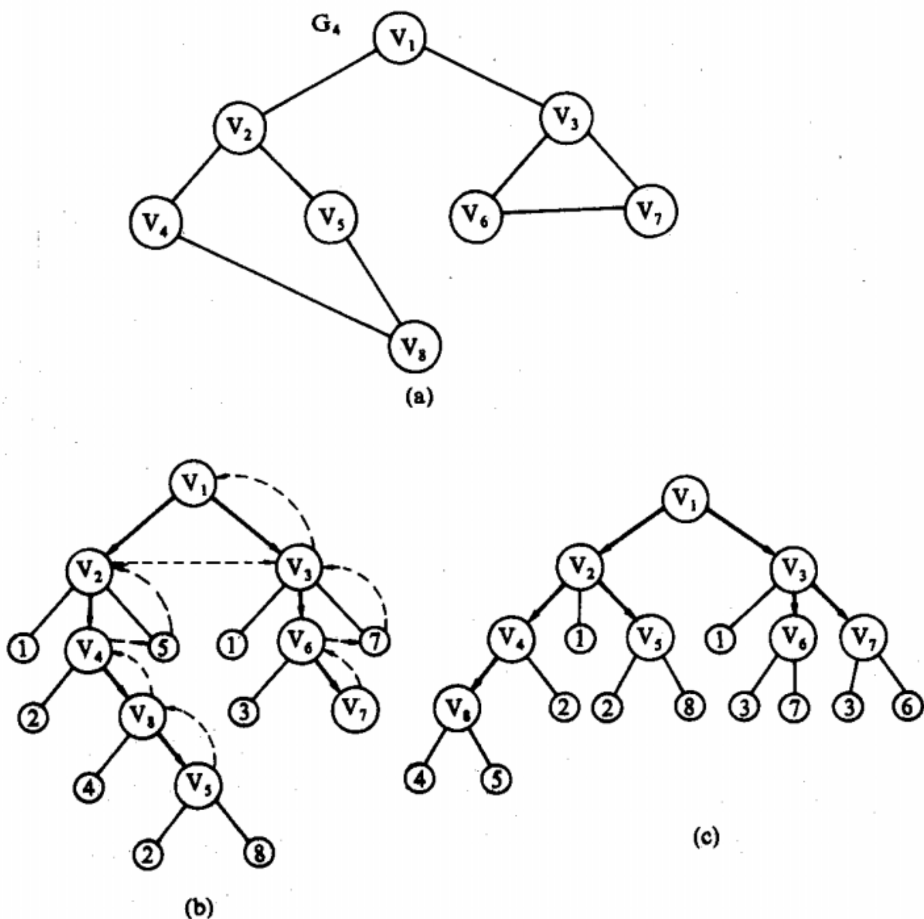
遍历图的过程
