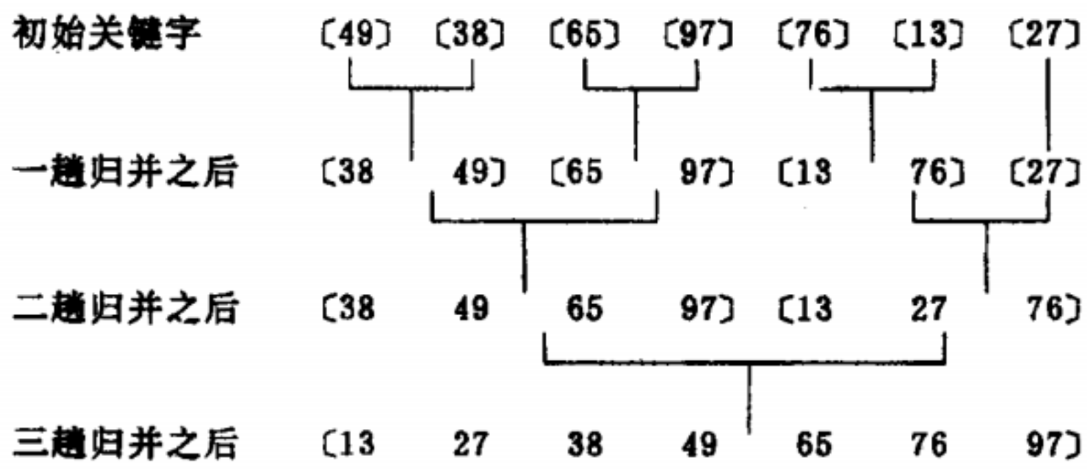
2—路归并排序的过程示例
