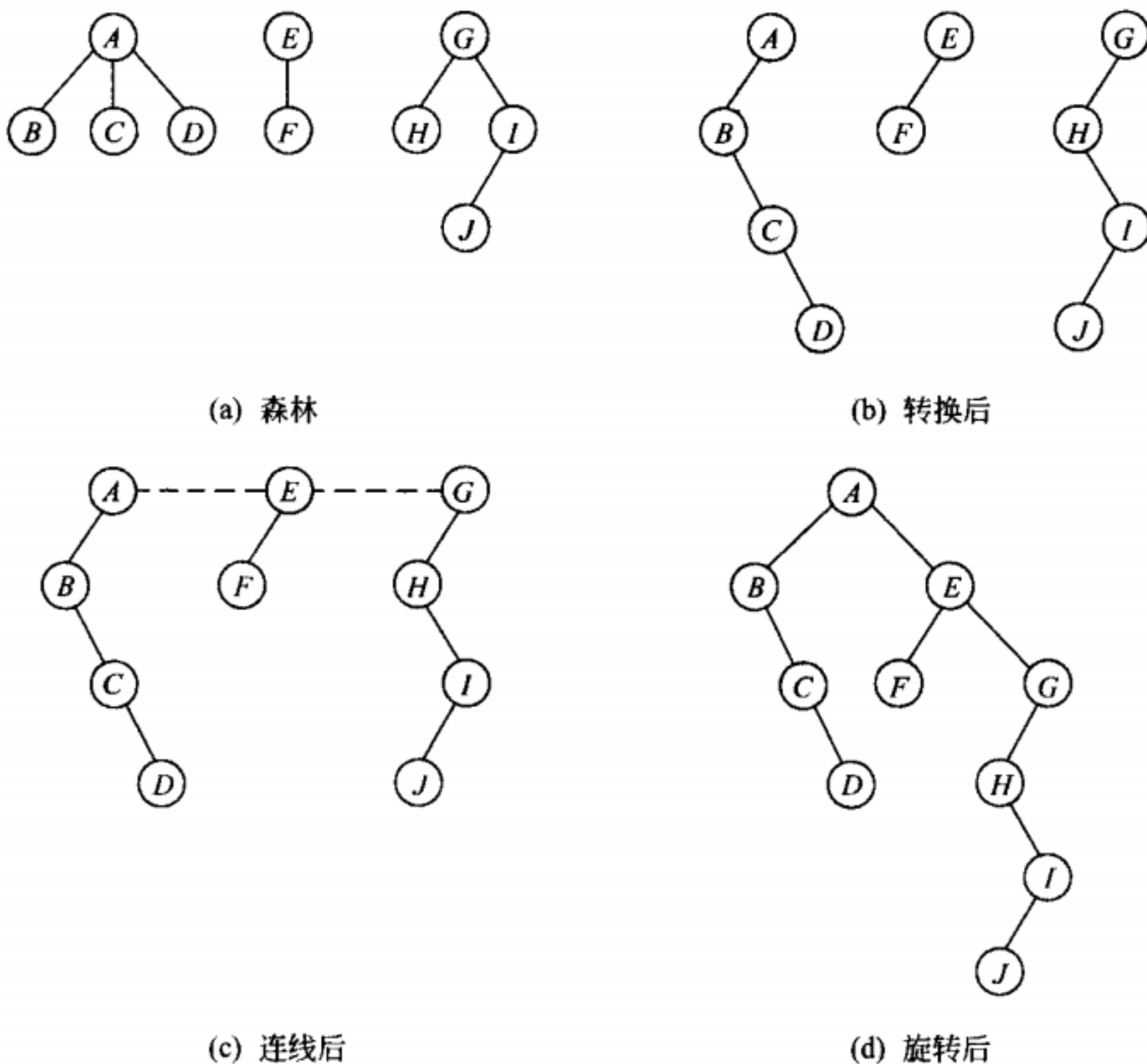
森林转换为二叉树的操作过程
