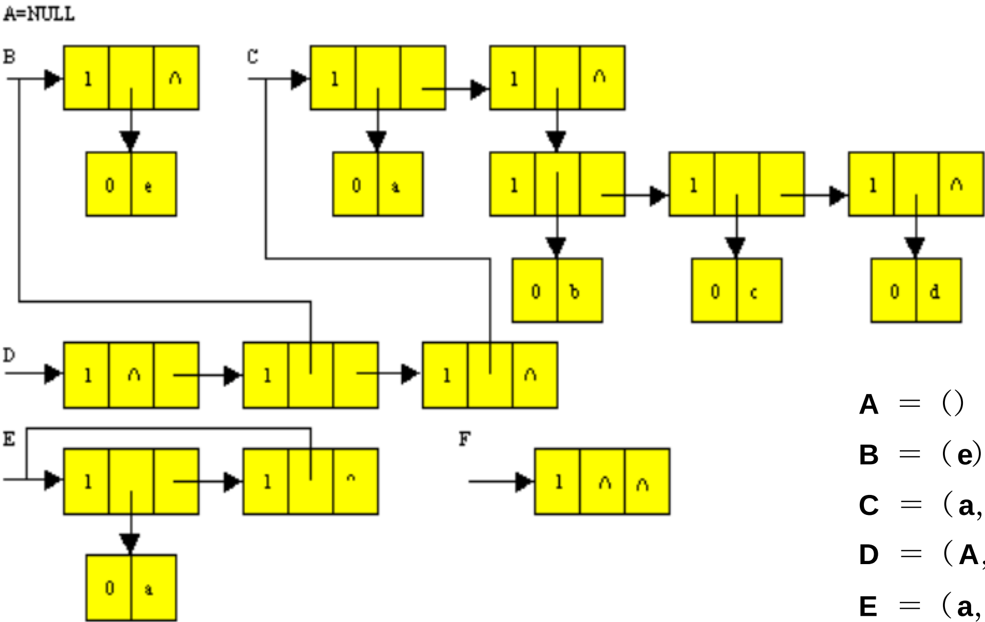
广义表的头尾表示法存储结构示例
