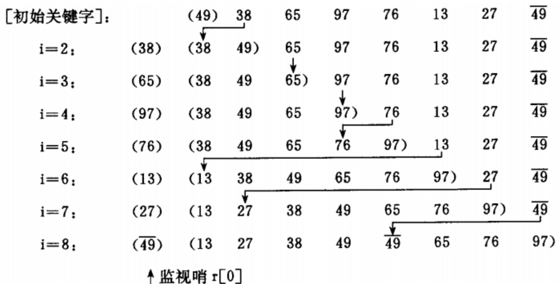
直接插入排序示例
