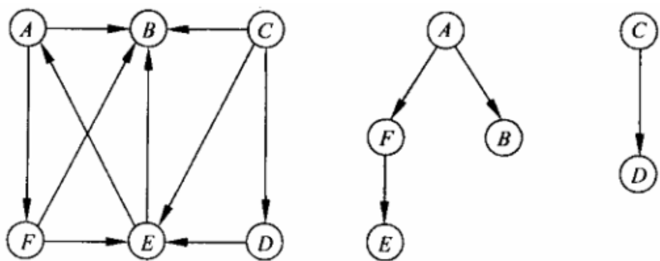
(a) 有向图 G_4
