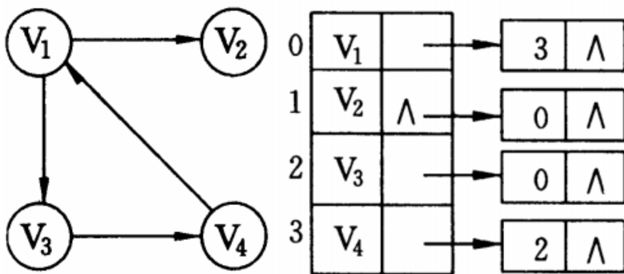
(a) 有向图 G1
