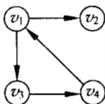
(a) 有向图 G1 及其他的邻接矩阵
