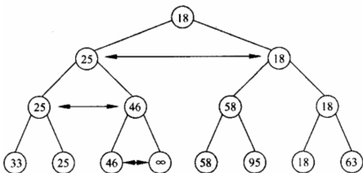
(b) 第二趟选择次小关键字过程示意
