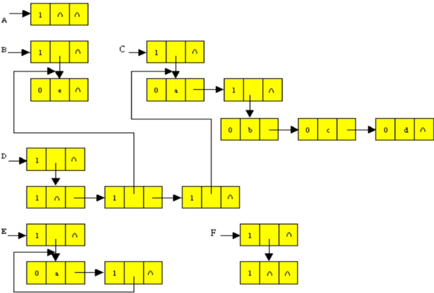
广义表的孩子兄弟表示法存储结构示例
