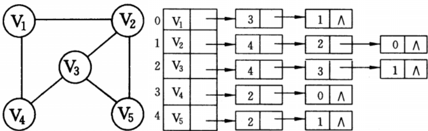
(a) 无向图 G2 及邻接表
