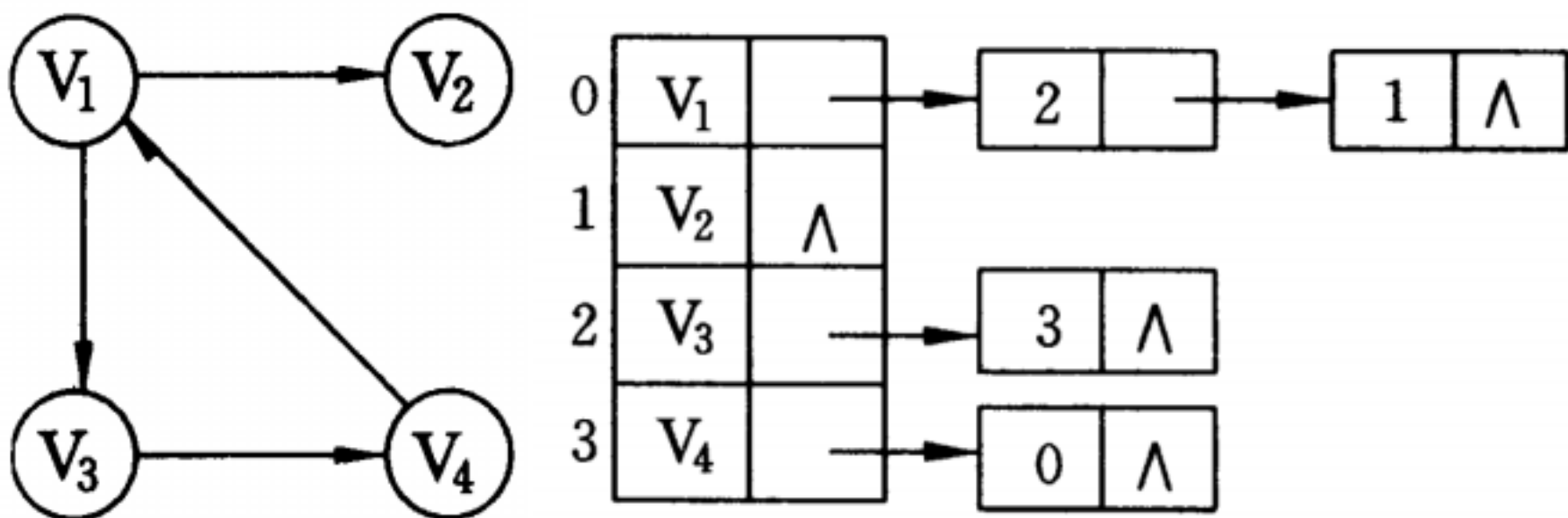
(b) 有向图 G1 及邻接表
