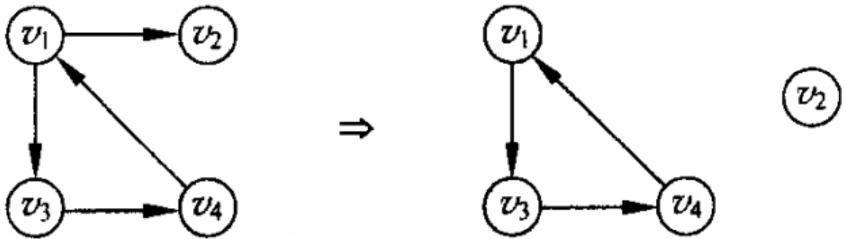
(a) 有向非连通图 G_1
