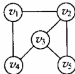
(b) 无向图 G2 及其他的邻接矩阵
