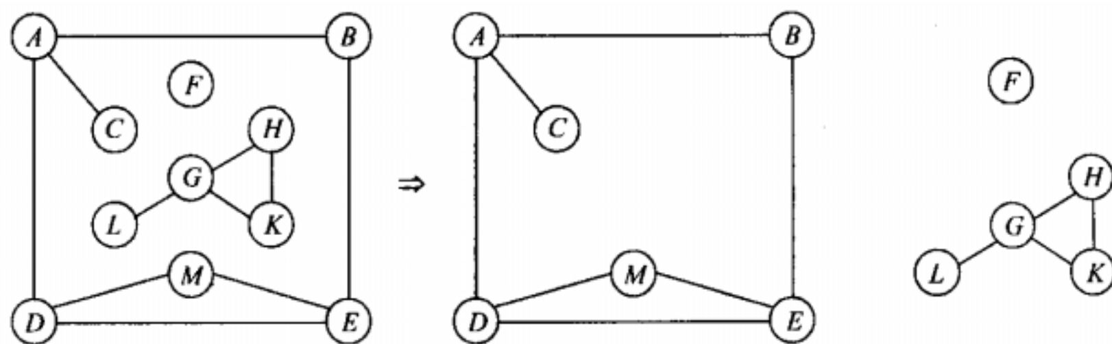
(a) 无向非连通图 G_3
