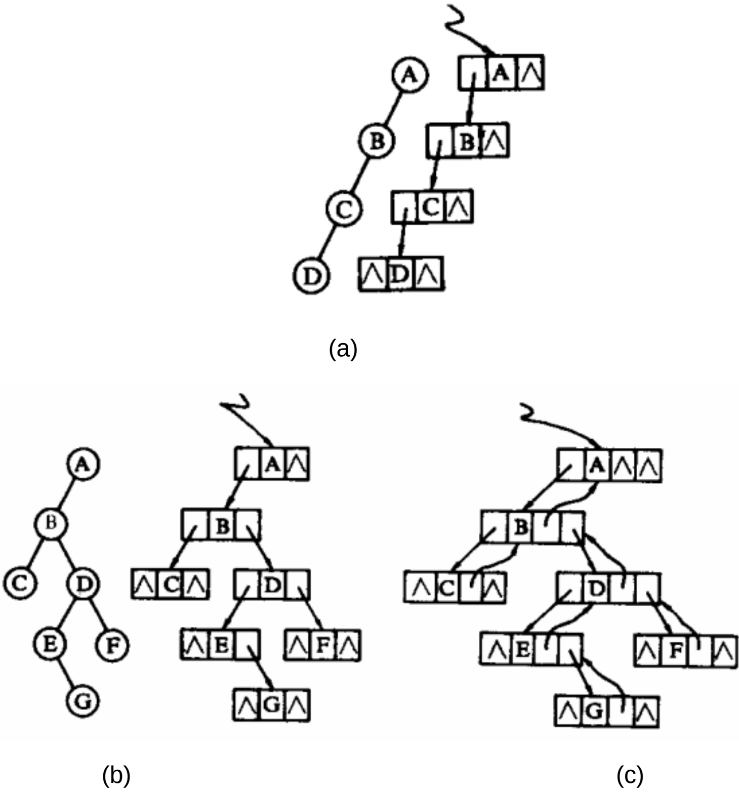
图 5.9 链表存储结构
