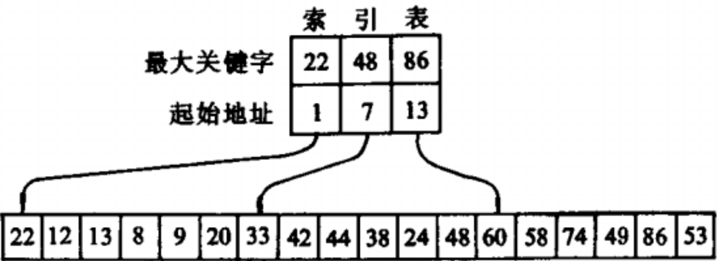
线性表及其索引表
